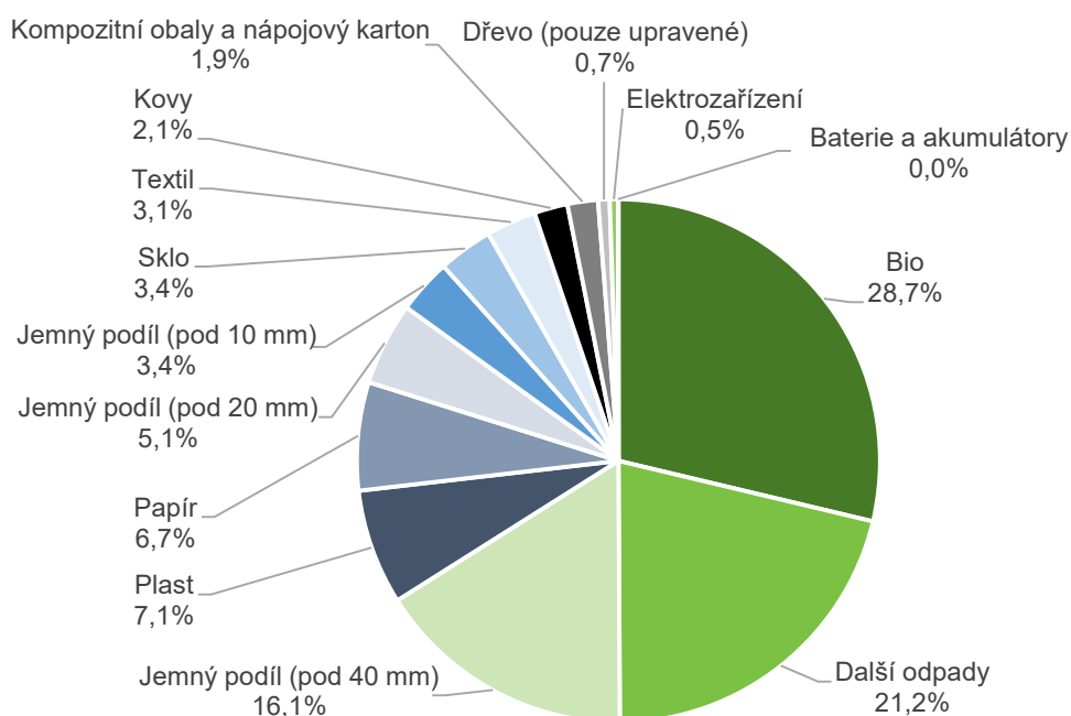
Graf 62: Průměrné složení SKO, hodnoty jsou uvedeny v % hm. 23
