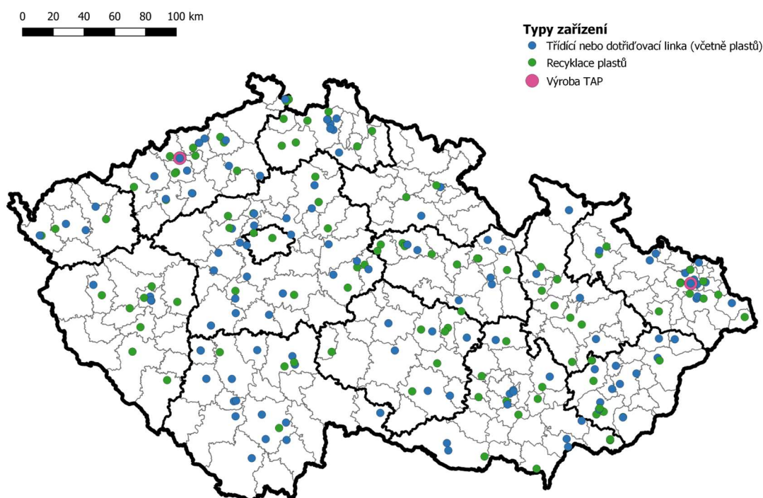
Obrázek 18: Mapa aktivních zařízení nakládajících s plastem označené jako třídící nebo dotřídovací linka, recyklace a výroba tuhých alternativních paliv
