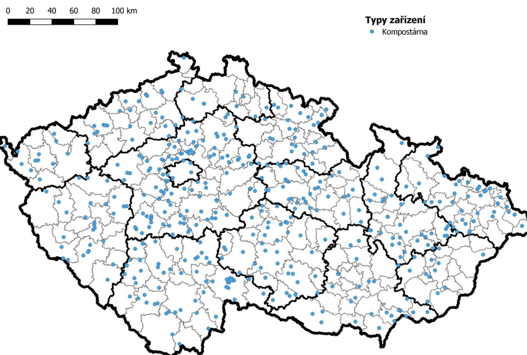
Obrázek 12: Mapa aktivních zařízení nakládajících s biologicky rozložitelným odpadem označené jako kompostárna
