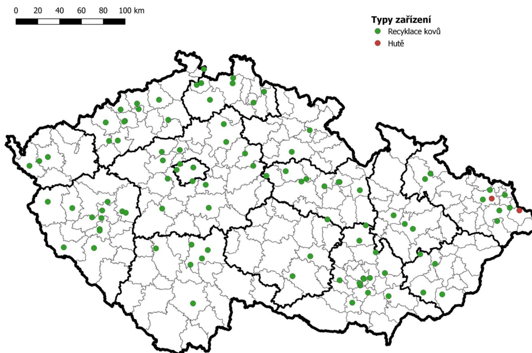
Obrázek 16: Mapa aktivních zařízení nakládajících s kovy označené jako hutě a recyklace kovů
