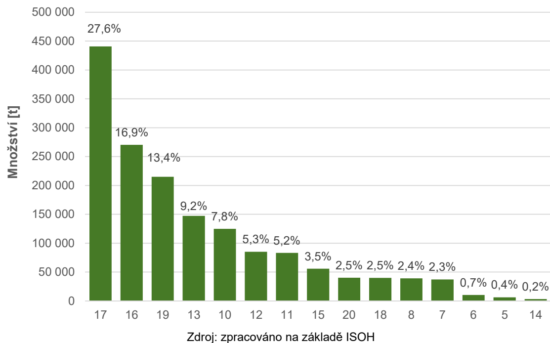
Graf 39: Skupiny katalogu odpadů zastoupené v nebezpečných odpadech v roce 2022 – top 15
