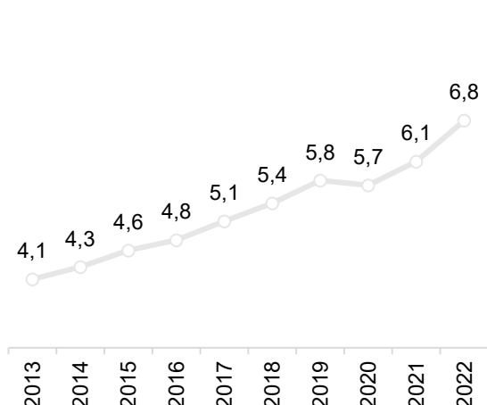
Graf 6: Vývoj HDP (bil. Kč, b.c.)
