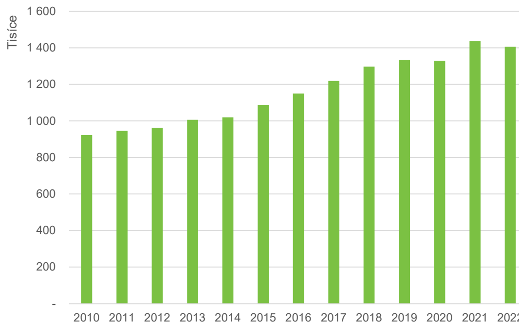
Graf 44: Celkové množství obalových odpadů, které vznikly v České republice mezi lety 2010 a 2022 v tisících tun:
