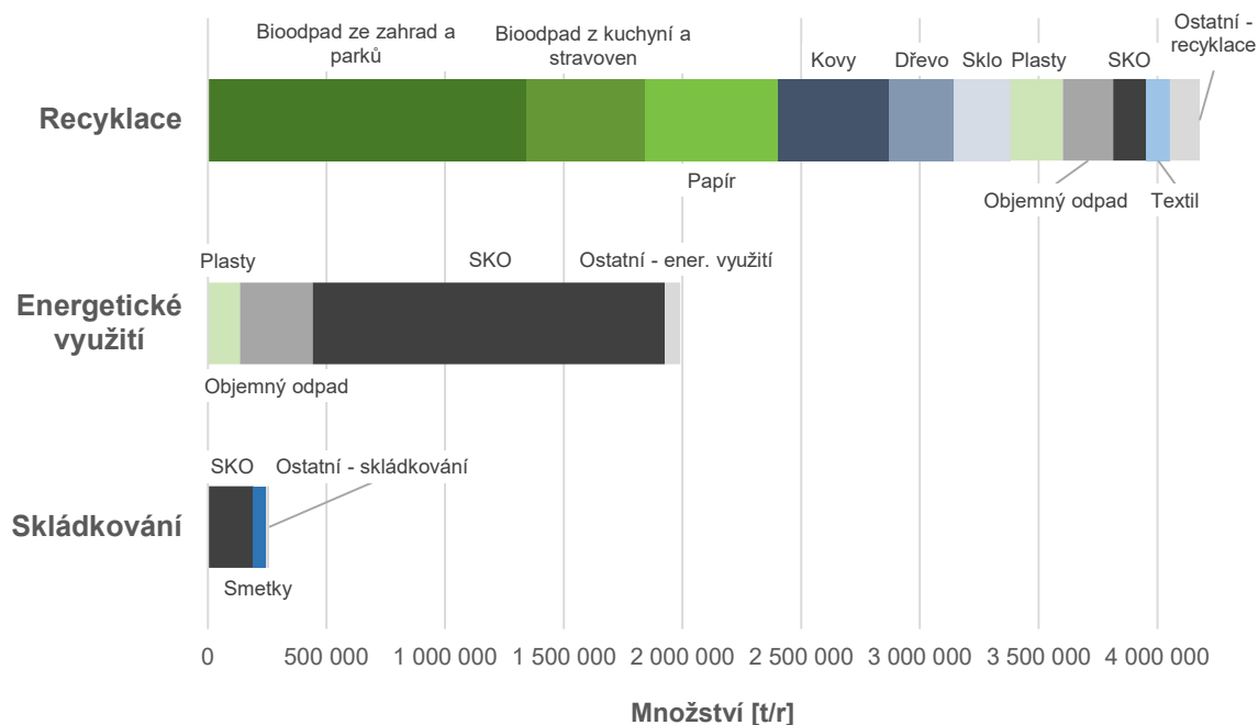
Graf 67: Příspěvky jednotlivých subtoků komunálního odpadu ke stěžejním způsobům nakládání v roce 2035 – scénář nakládání N2 (skládování 5 % produkce komunálních odpadů)
