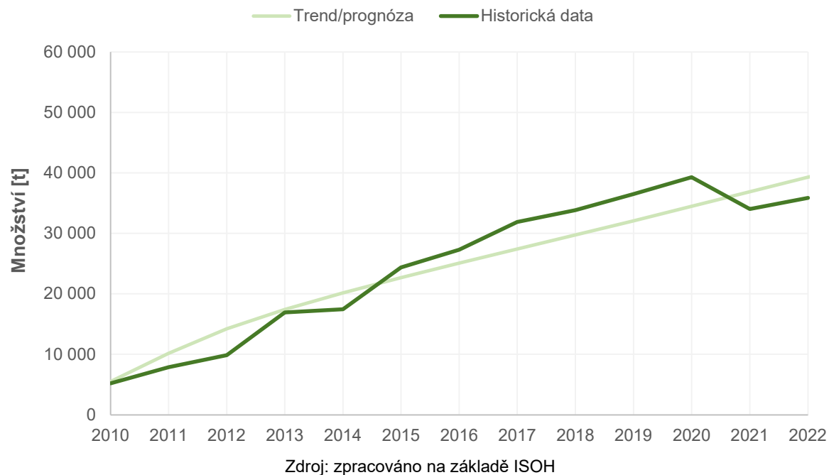
Graf 24: Vývoj produkce textilu z odděleného soustředování (skupina 20)
