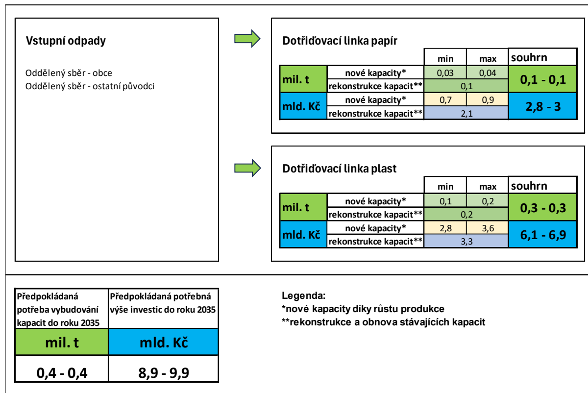
Obrázek 30: Předpokládané investice do technologií k zajištění úpravy odpadu z odděleného sběru využitelných odpadů (papír, plast)
