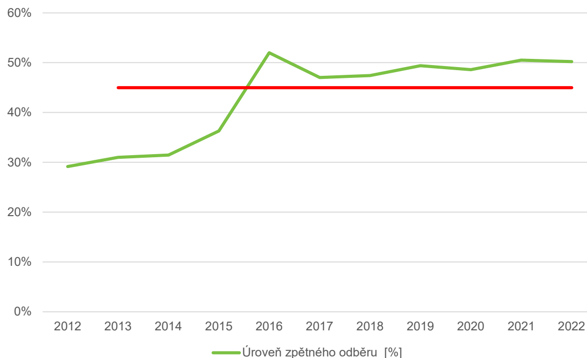
Graf 41: Vývoj úrovně zpětného odběru odpadních baterií v České republice mezi lety 2012 a 2022
