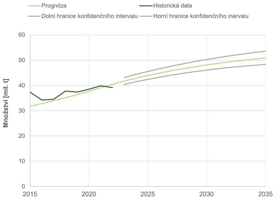
Graf 61: Prognóza vývoje produkce všech odpadů do roku 2035
