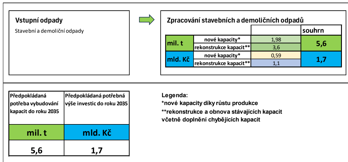
Obrázek 33: Předpokládané investice do technologií pro nakládání se stavebními a demoličními odpady
