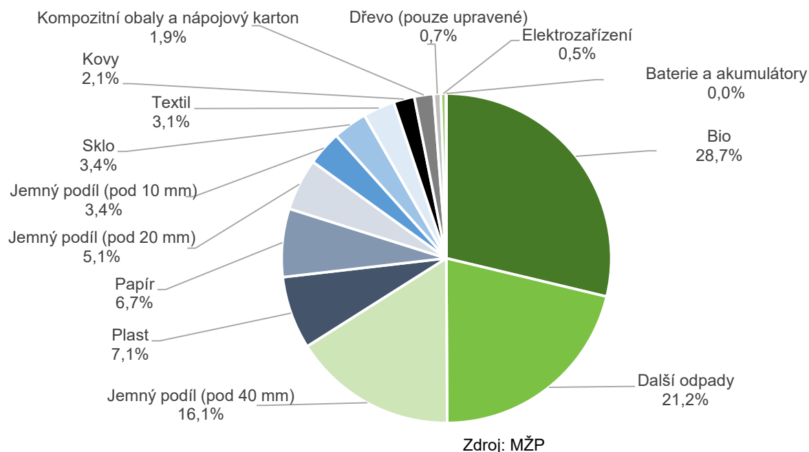
Graf 33: Průměrné složení SKO v ČR, hodnoty jsou uvedeny v % hm. 23
