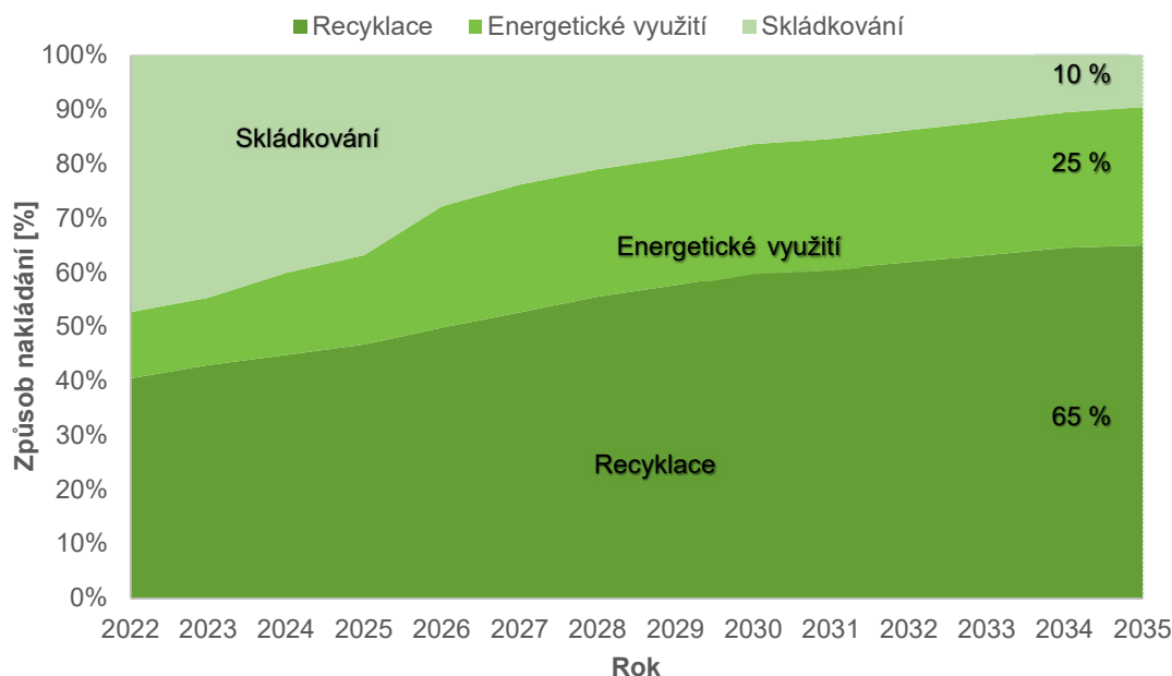
Graf 64: Model nakládání s komunálními odpady pro scénář nakládání N1 (graf společný pro optimistický i realistický scénář produkce komunálního odpadu – trajektorie T1 a T2)
