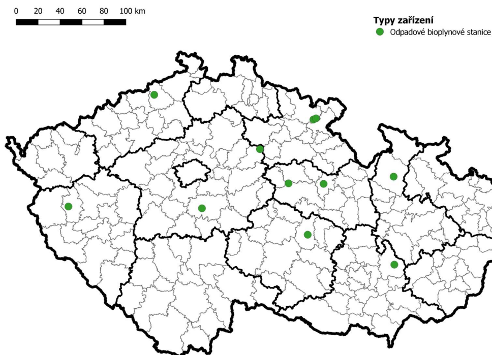
Obrázek 13: Mapa aktivních zařízení nakládajících s biologicky rozložitelným odpadem označené jako bioplynové stanice
