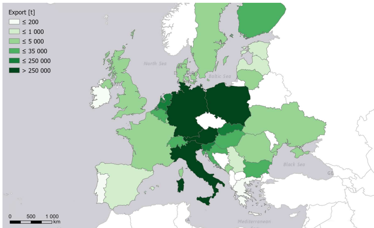
Obrázek 28: Mapa států, kam probíhal export odpadu z ČR v roce 2022 – Evropa
