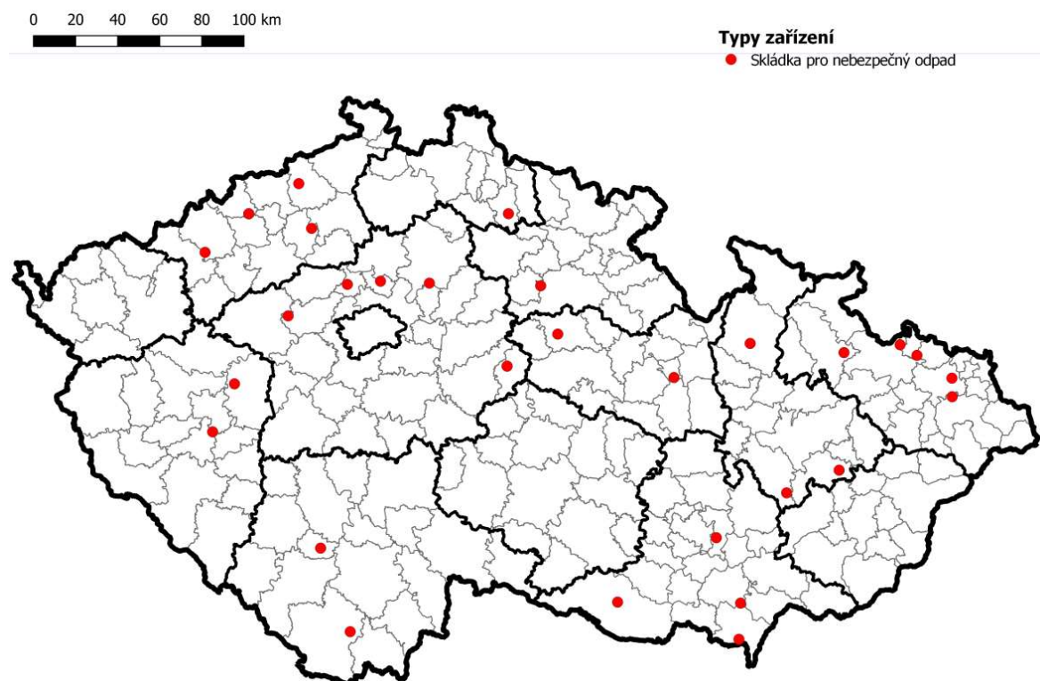
Obrázek 23: Mapa skládek pro nebezpečný odpad (S-NO)
