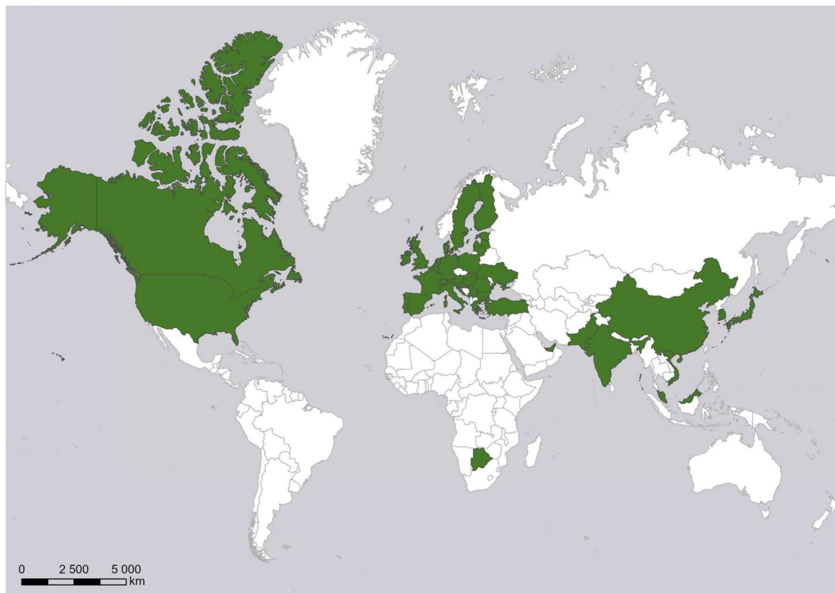
Obrázek 27: Mapa států, kam probíhal export odpadu z ČR v roce 2022
