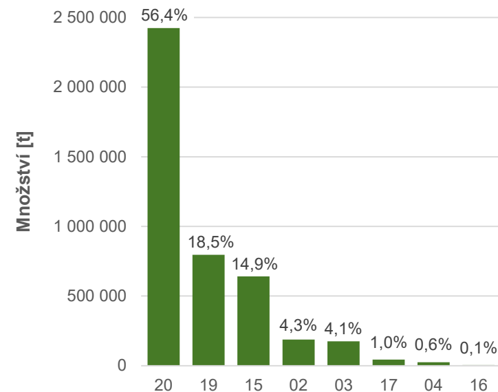
Graf 48: Produkce biologicky rozložitelného odpadu v roce 2022 dle skupin odpadů
