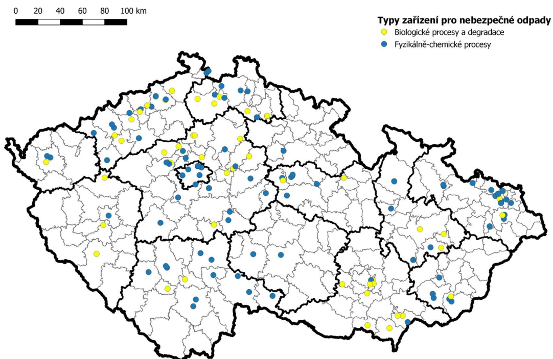
Obrázek 20: Mapa aktivních zařízení nakládajících s nebezpečným odpadem označené jako biologické procesy a degradace a fyzikálně-chemické procesy
