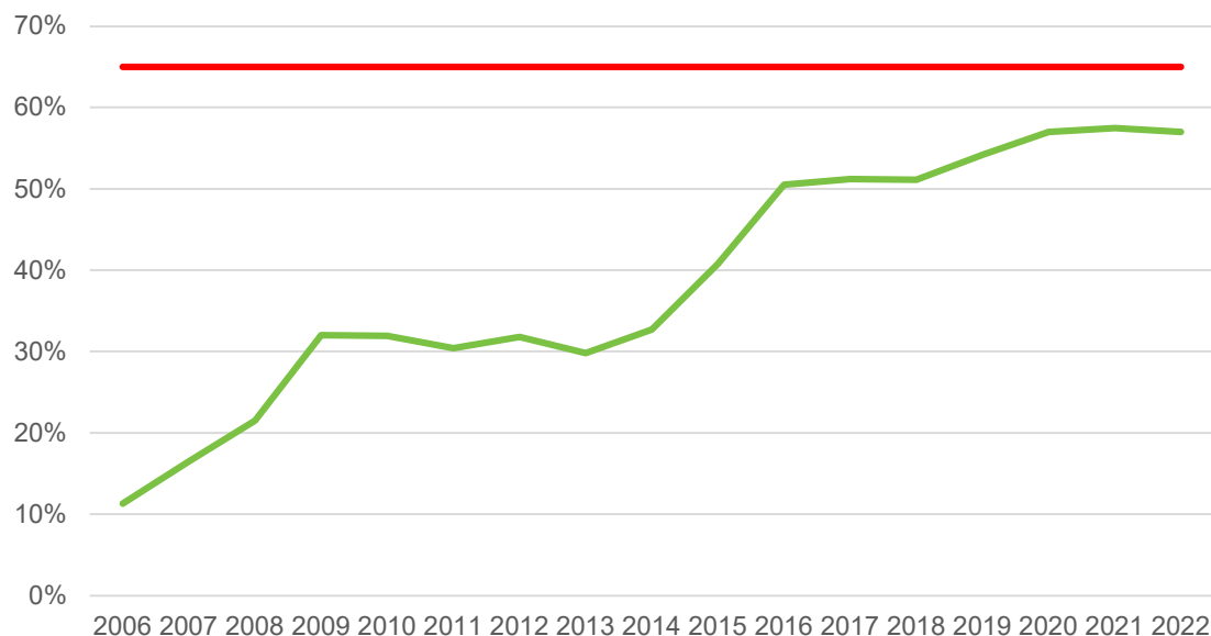
Graf 40: Vývoj úrovně zpětného odběru odpadních elektrozařízení v České republice mezi lety 2006 a 2022
