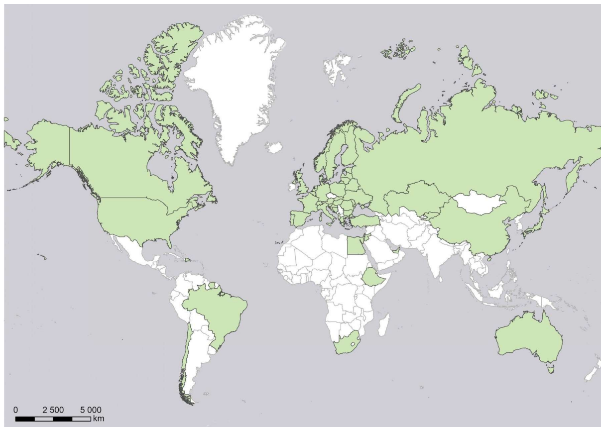
Obrázek 25: Mapa států odkud probíhal import odpadu do ČR v roce 2022
