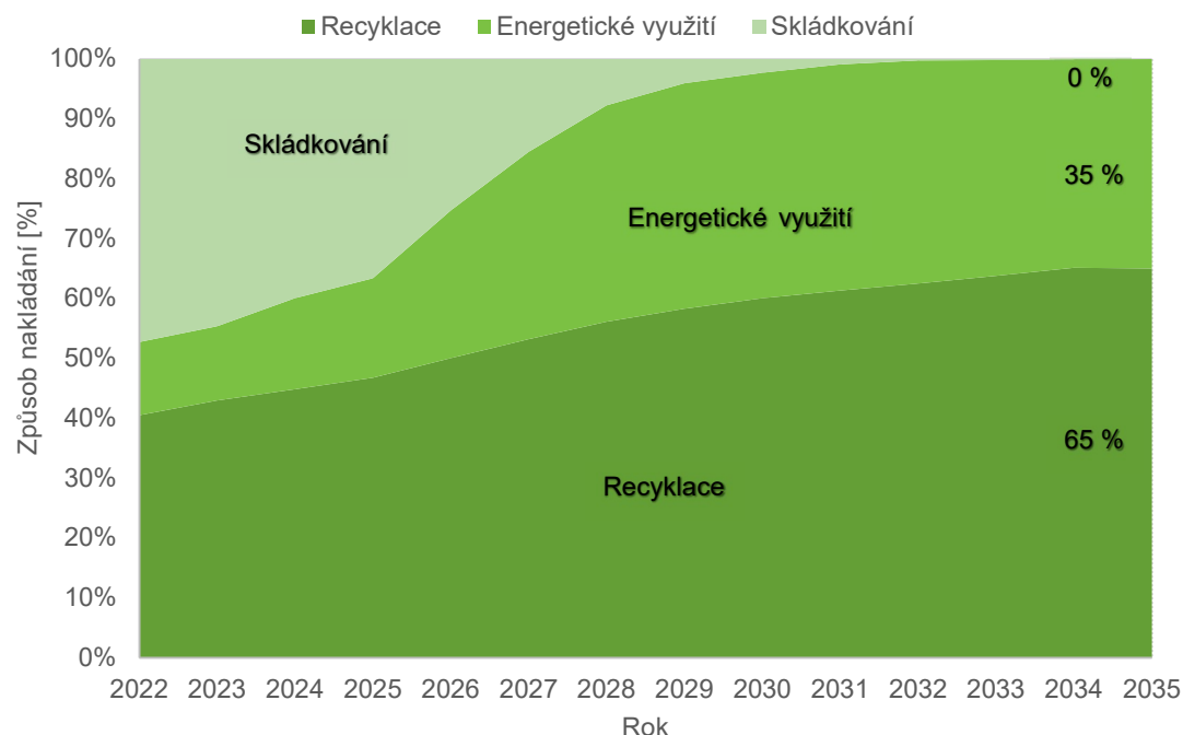
Graf 66: Model nakládání s komunálními odpady pro scénář nakládání N3 (graf společný pro optimistický i realistický scénář produkce komunálního odpadu – trajektorie 1 a 2)
