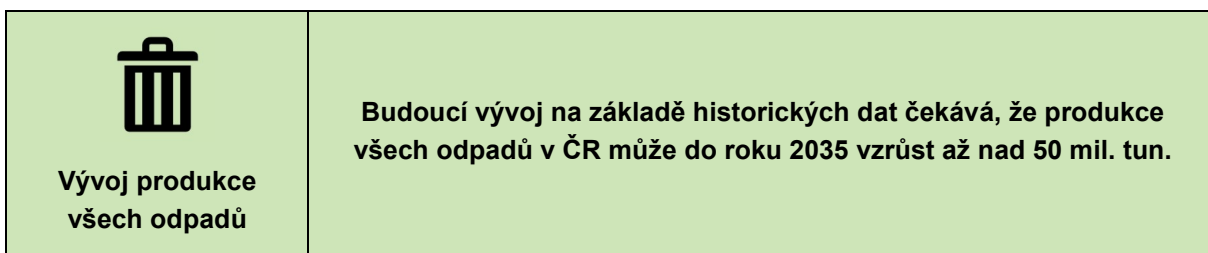
Graf 61: Prognóza vývoje produkce všech odpadů do roku 2035
