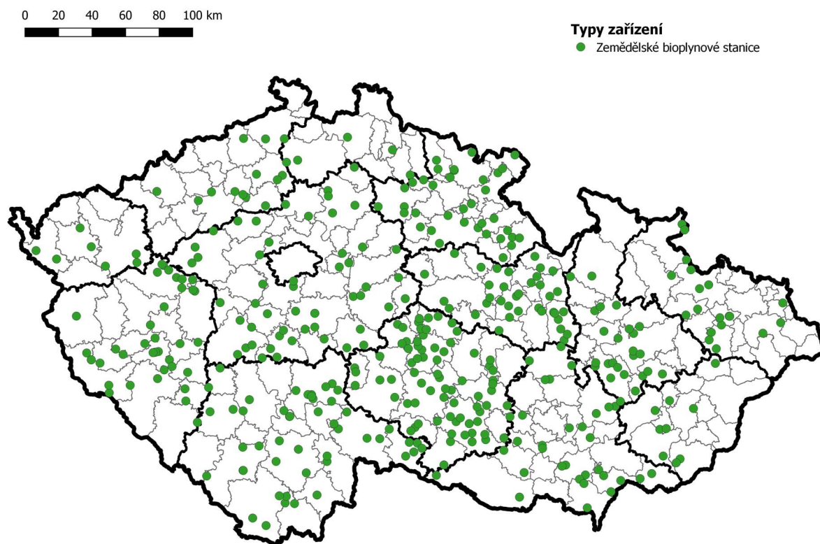
Obrázek 14: Mapa zemědělských bioplynových stanic
