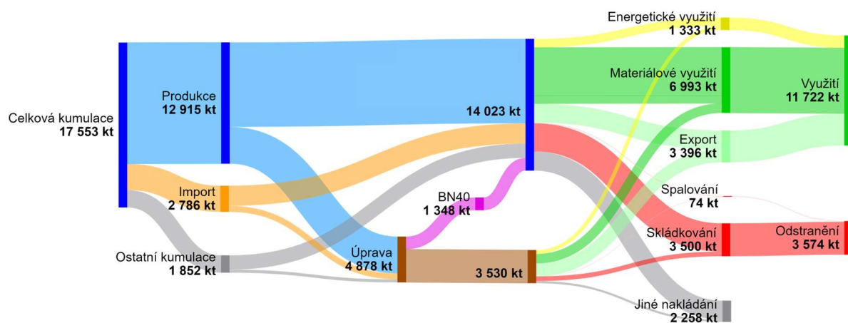
Graf 12: Znázornění toku odpadů v ČR v roce 2022 – Celková produkce odpadů bez minerálních odpadů
