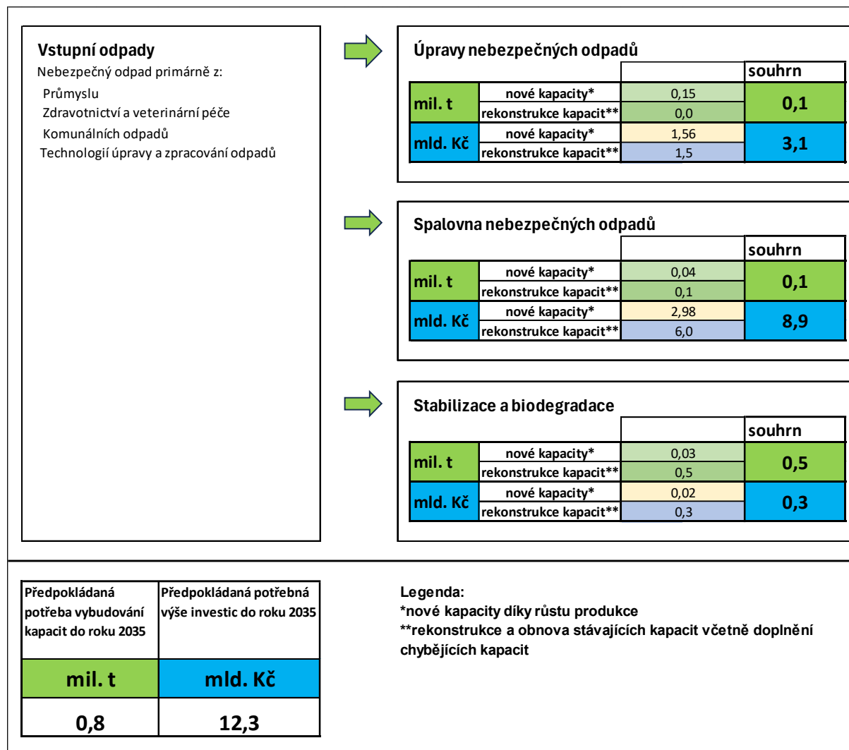
Obrázek 32: Předpokládané investice do technologií pro nakládání s nebezpečnými odpady
