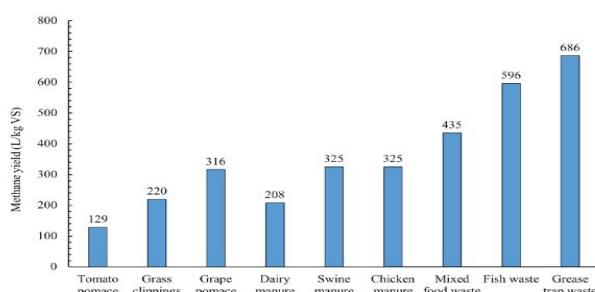
Obrázek 4-14 Výtěžnost metanu z různých organických odpadů
