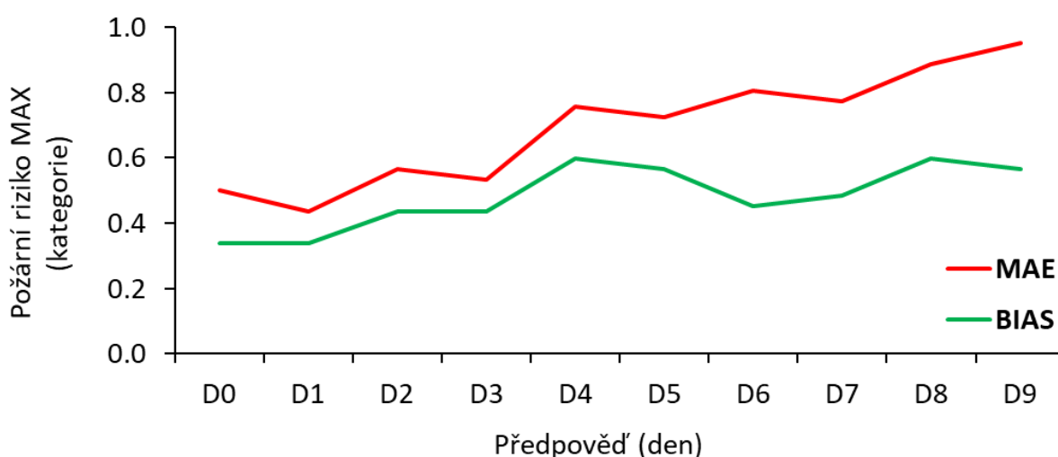
Obr. 59 Absolutní chyba (MAE) a odchylka (BIAS) předpovědi maximálního požárního rizika (souhrnný index) na daný den (D0) až 9 dnů dopředu (D9) pro zkoumanou oblast v období 1.7.–31.8.2022.
