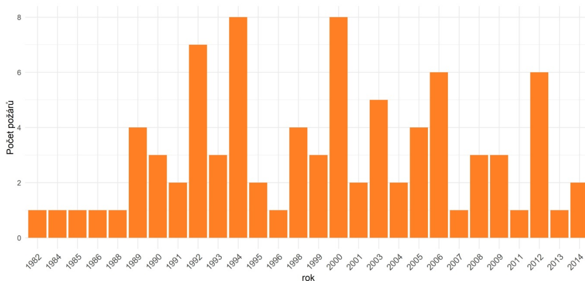
Obr. 3b Počet požárů na území NP České Švýcarsko v období 1982-2014.
