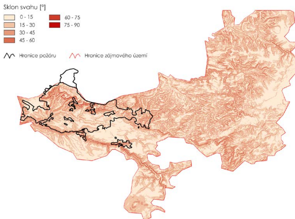
Obr. 68 Vstupní vrstva do programu FlamMap v rozlišení 5 x 5 m, sklon svahu
