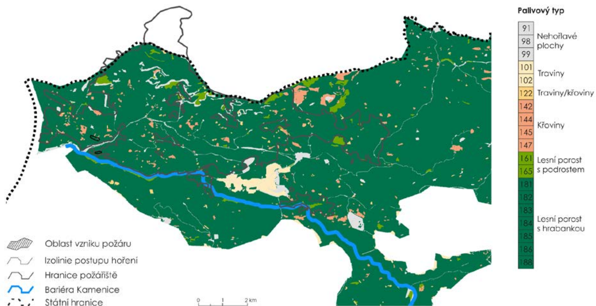
Obr. 79 Vstupní vrstva do programu FlamMap v rozlišení 5 × 5 m, palivové typy pro scénář 5
