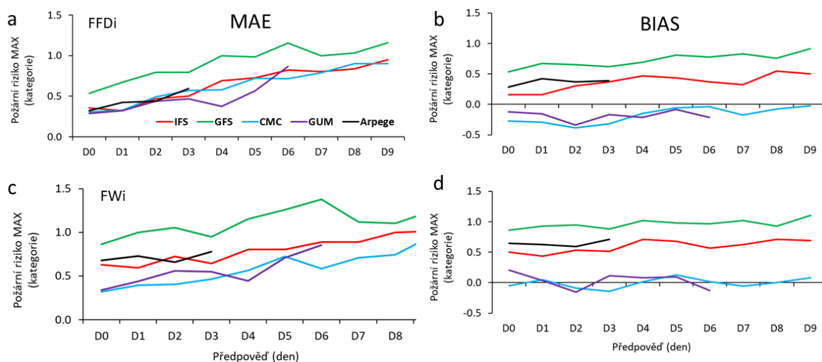
Obr. 65 Absolutní chyba (MAE) a odchylka (BIAS) předpovědi maximálního požárního rizika podle dvou požárních indexů a 5 numerických předpovědních modelů na daný den (D0) až 9 dnů dopředu (D9) pro zkoumanou oblast v období 1.7.–31.8.2022.
