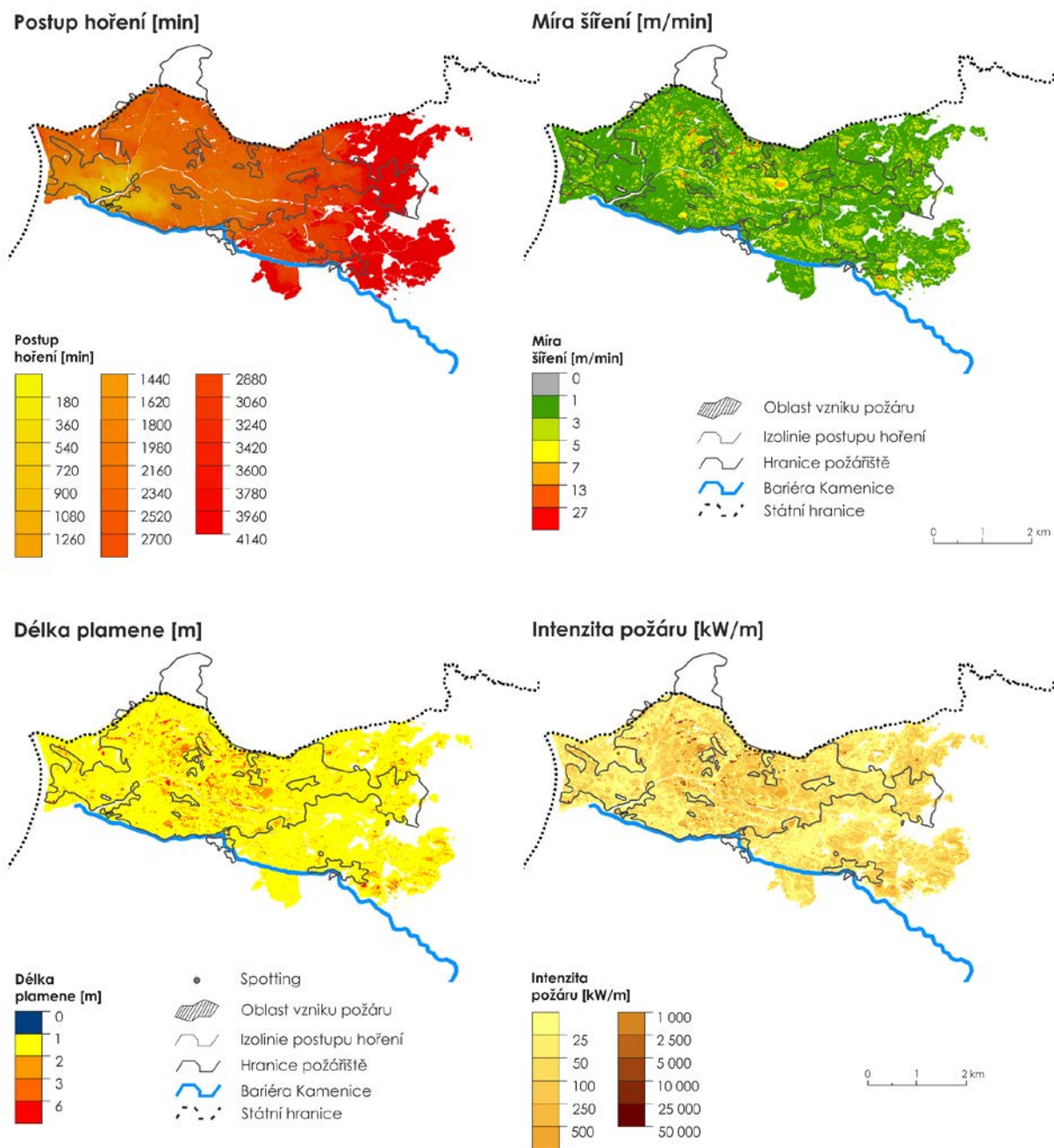
Obr. 76 Simulace požáru, kdy došlo ke snížení teploty o 50 % oproti naměřené teplotě na meteorologické stanici Tokaň, veškeré další parametry zůstaly stejné jako ve scénáři 1.
