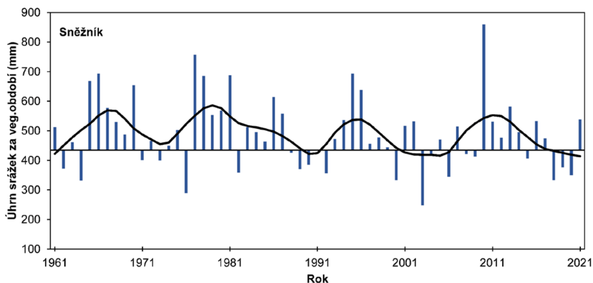
Obr. 42 Kolísání úhrnů srážek za duben až září vyjádřené odchylkami od normálu 1991 až 2020 na stanicích Děčín a Sněžník. Shlazeno Gaussovým filtrem pro 10 let.
