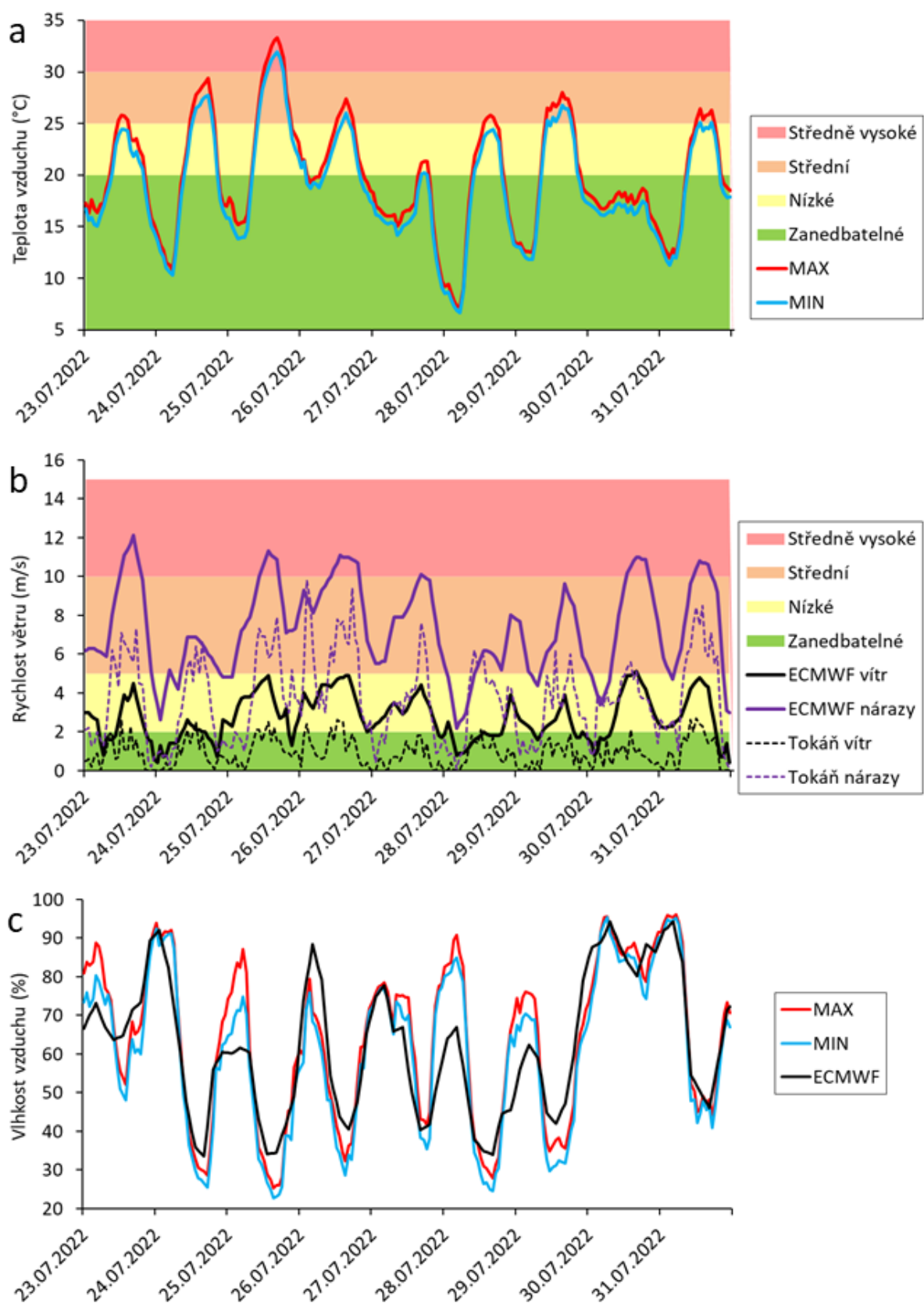
Obr. 45 Prostorový hodinový průměr teploty vzduchu na základě meteorologických stanic (a); průměrná hodinová rychlost větru a maximální hodinové nárazy větru podle modelu ECMWF IFS a ze stanice Tokáň (b); relativní vlhkost vzduchu jako prostorový hodinový průměr na základě
