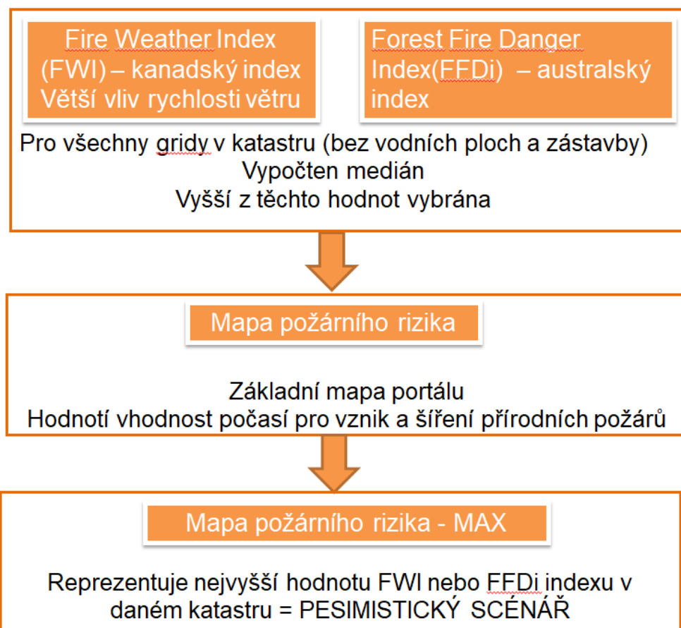
Obr. 52 Schéma výpočtu požárního rizika na základě dvou požárních indexů, jak je zobrazeno na portálu www.firerisk.cz
