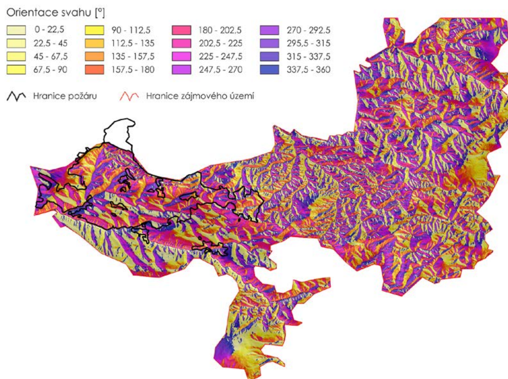
Obr. 69 Vstupní vrstva do programu FlamMap v rozlišení 5 x 5 m, orientace svahu
