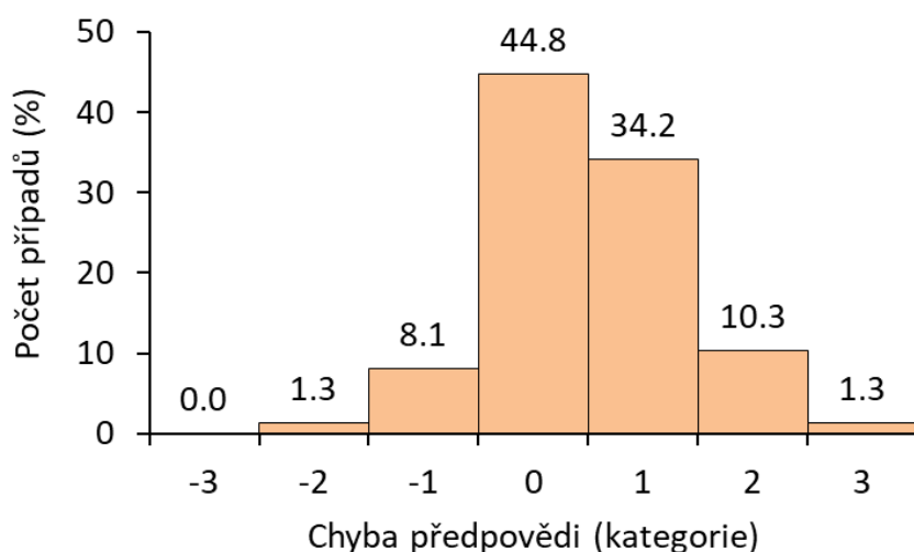
Obr. 61 Histogram rozdílu předpovědi maximálního požárního rizika (souhrnný index) a skutečnosti pro jednotlivé dny za období 1.7.–31.8.2022
