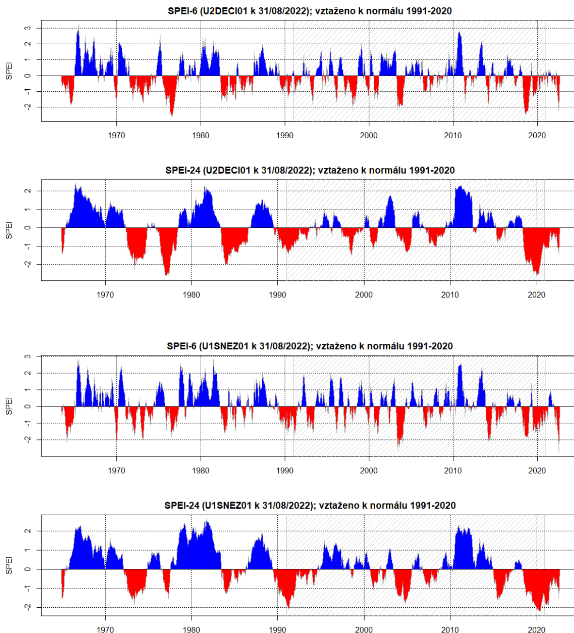
Obr. 43 Kolísání indexů SPEI-6 a SPEI-24 na stanici Děčín a Sněžník za posledních 60 let.
