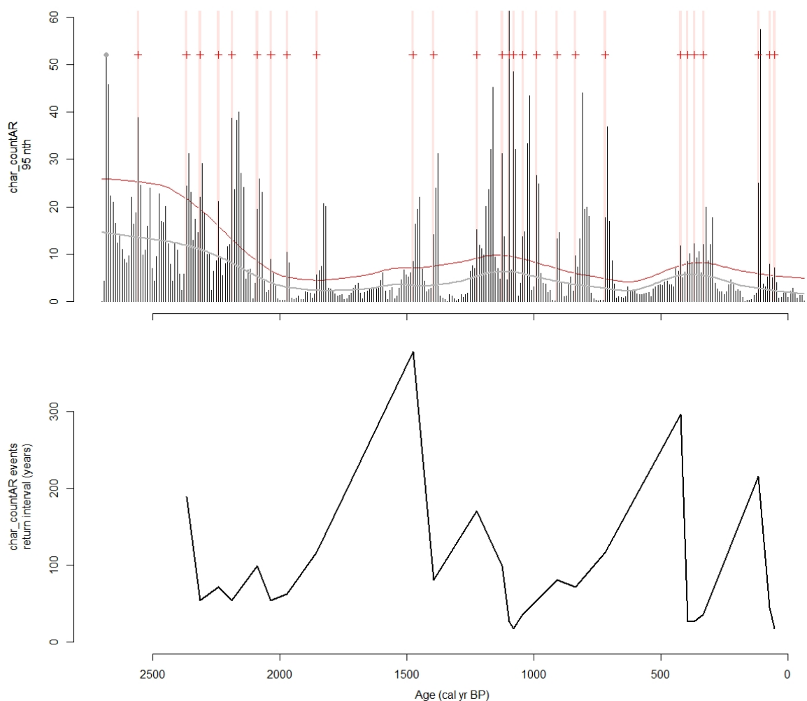
Obr. 7 Požárová historie na lokalitě Pravčický důl. Horní panel – sloupcový graf množství depozice uhlíků do sedimentu (CHAR), červená křivka představuje dlouhodobý trend, křížky označují statisticky významné požárové události. Spodní panel – interval návratu požáru (fire return interval, FRI). Nepublikováno.
