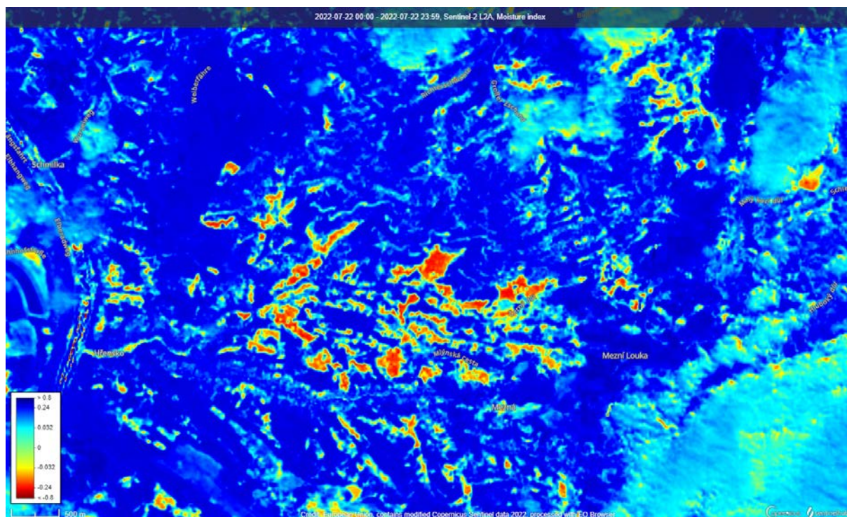
Obr. 51 Vlhkostní index získaný družicí Sentinel 2 dne 22. července 2022.
