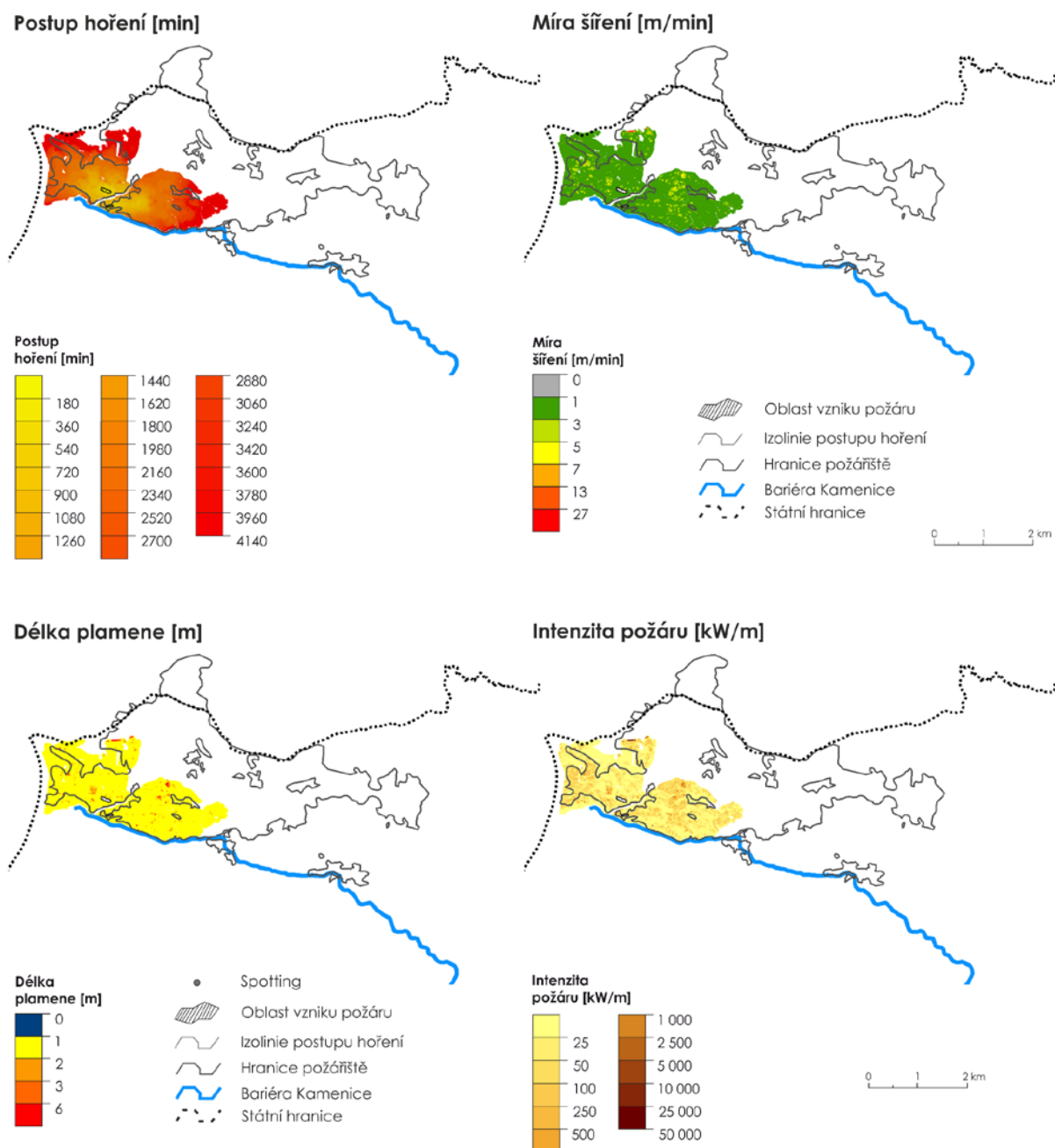
Obr. 74 Postup hoření a míra šíření za změněných podmínek větru (naměřené nárazy větru a příslušný směr na meteorologické stanici Tokáň)
