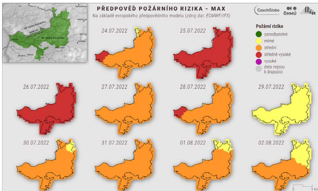
Obr. 56 Zachycuje hodnoty požárního rizika na základě dat portálu FireRisk se zjevným výrazným zhoršením hodnot ve dnech 25. a 26. července.
