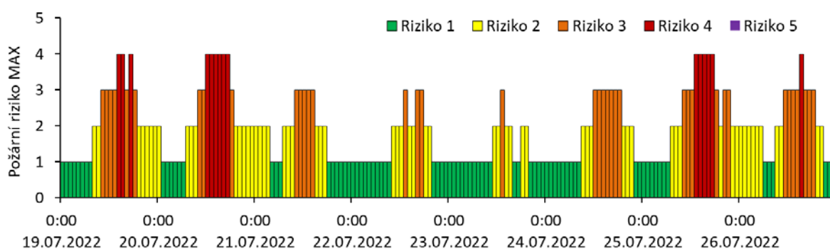
Obr. 54 Maximální požární riziko vyskytující se ve zkoumané oblasti jako souhrnný index pro jednotlivé hodiny v období 19.7.2022 až 26.7.2022
