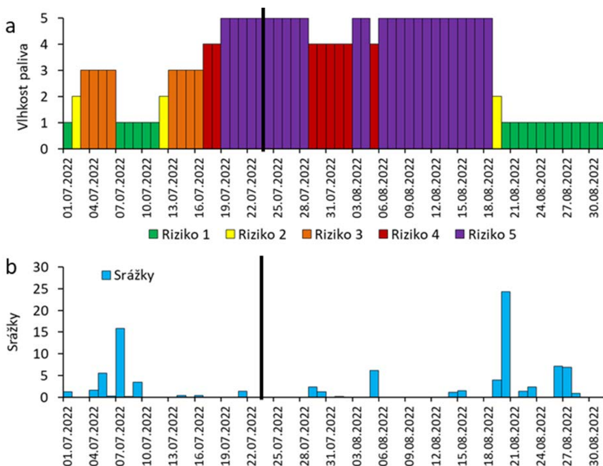
Obr. 46 Maximální hodnota rizika na základě vlhkosti paliva (a) a denní srážkové úhrny (b) na zkoumaném území v období 1.7.-31.8.2022 (Riziko 1 – zanedbatelné; Riziko 2 – nízké; Riziko 3 – střední; Riziko 4 – středně vysoké; Riziko 5 - vysoké)
