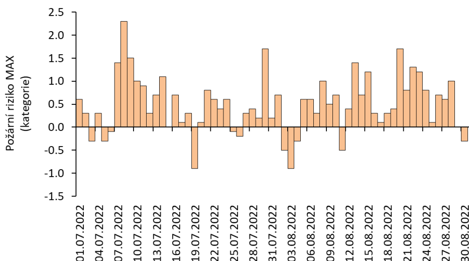
Obr. 60. Odchylka (BIAS) předpovědi maximálního požárního rizika (souhrnný index za všechny délky D0 až D9) pro jednotlivé dny za období 1.7.–31.8.2022
