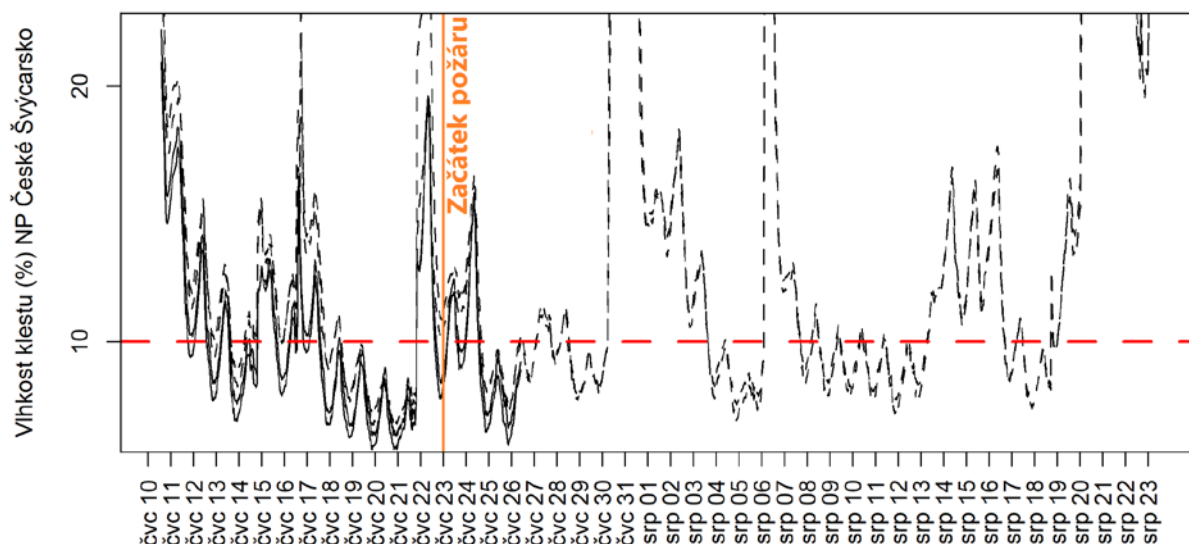
Obr. 48 Data vlhkosti paliva ze stanic FireRisk.cz z oblasti NP České Švýcarsko jak pro období 1.1. 2022-24.11. 2022 (nahore) tak detailní výřez pro období těsně před a během požáru (dole). Pozn. Dne 26.8. zničil postupující požár jednu ze stanic.
