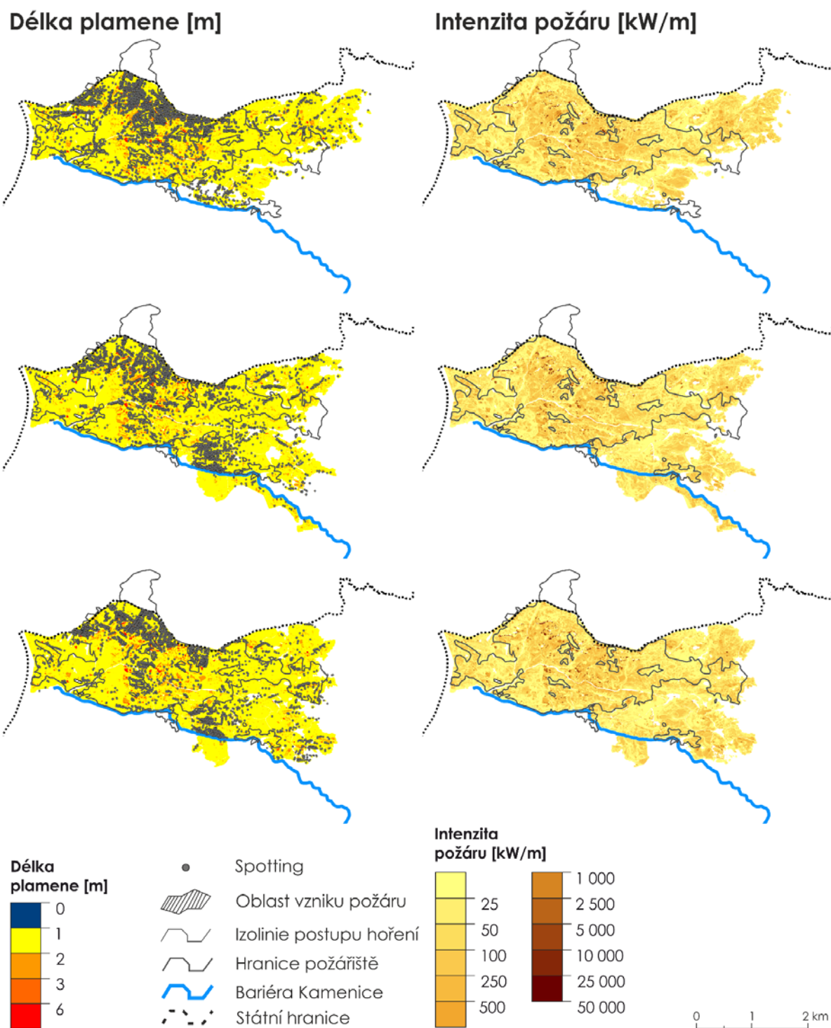
Obr. 72 Ukázka tří simulací reflektující reálný postup požáru za aktuálně dostupných informací, a to na příkladu charakteristiky požáru Délka plamene a Intenzita požáru
