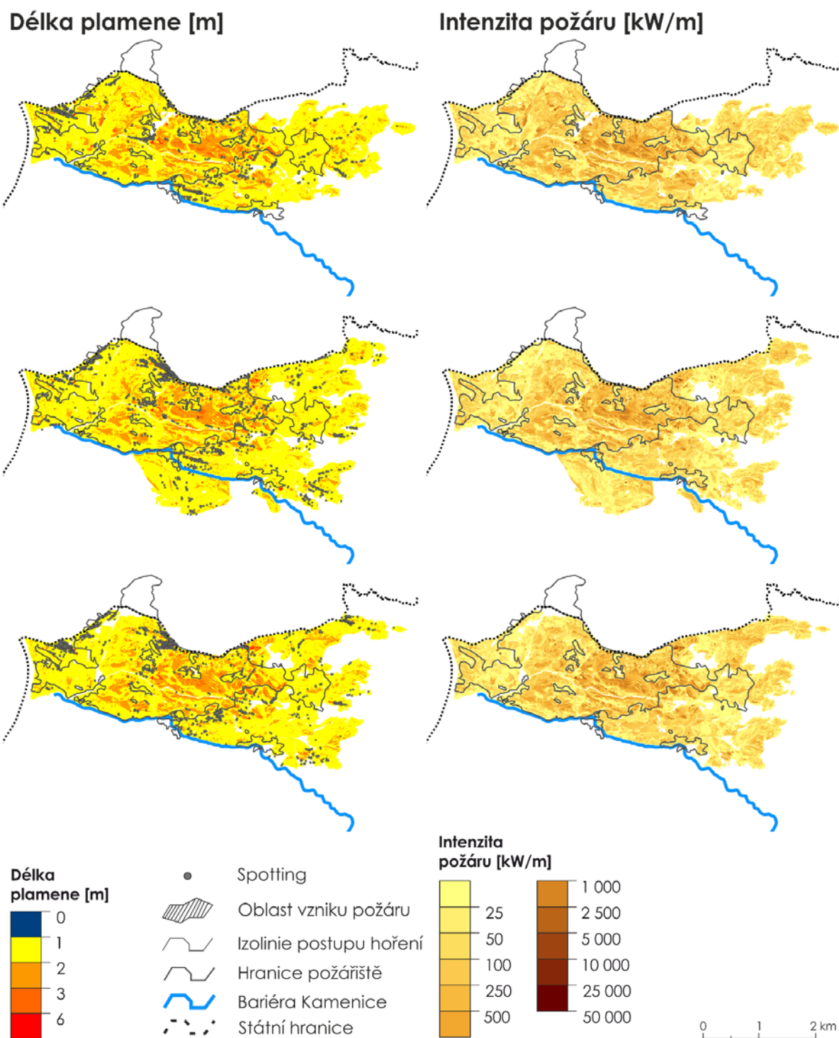
Obr.84 Ukázka tří simulací představující požár v holinách, Délka Plamene a Intenzita požáru
