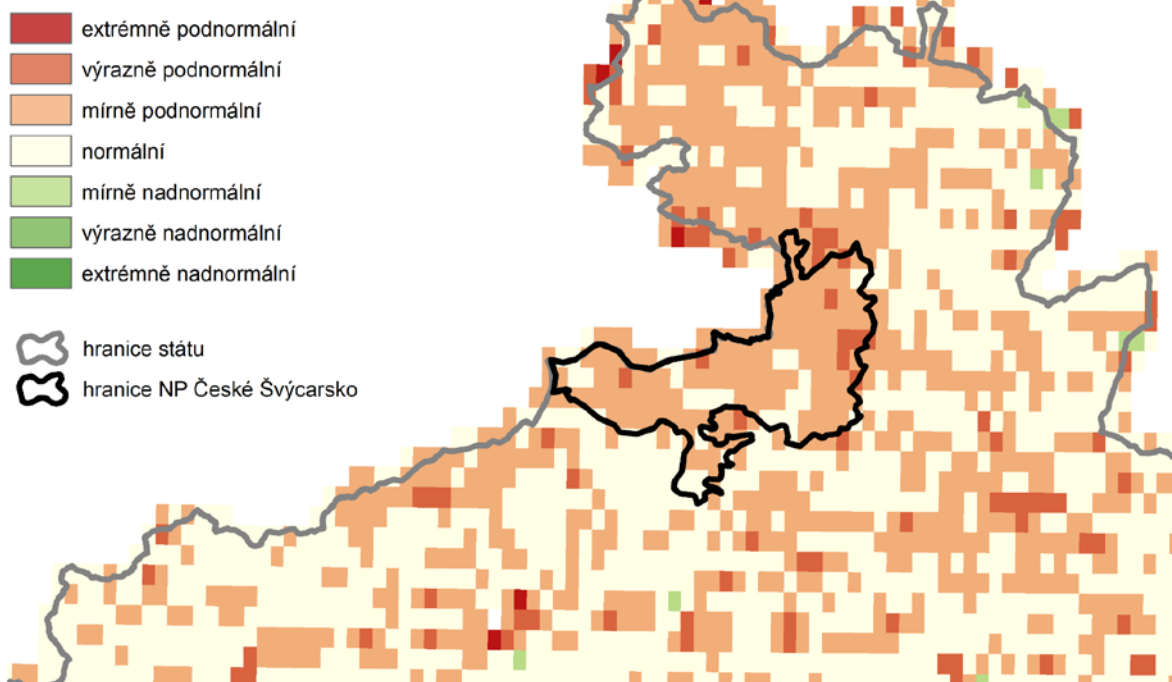
Obr. 49 Anomálie vegetace podle satelitem měřeného FAPAR (frakce absorbovaného fotosynteticky aktivního záření) v březnu až červenci 2022.
