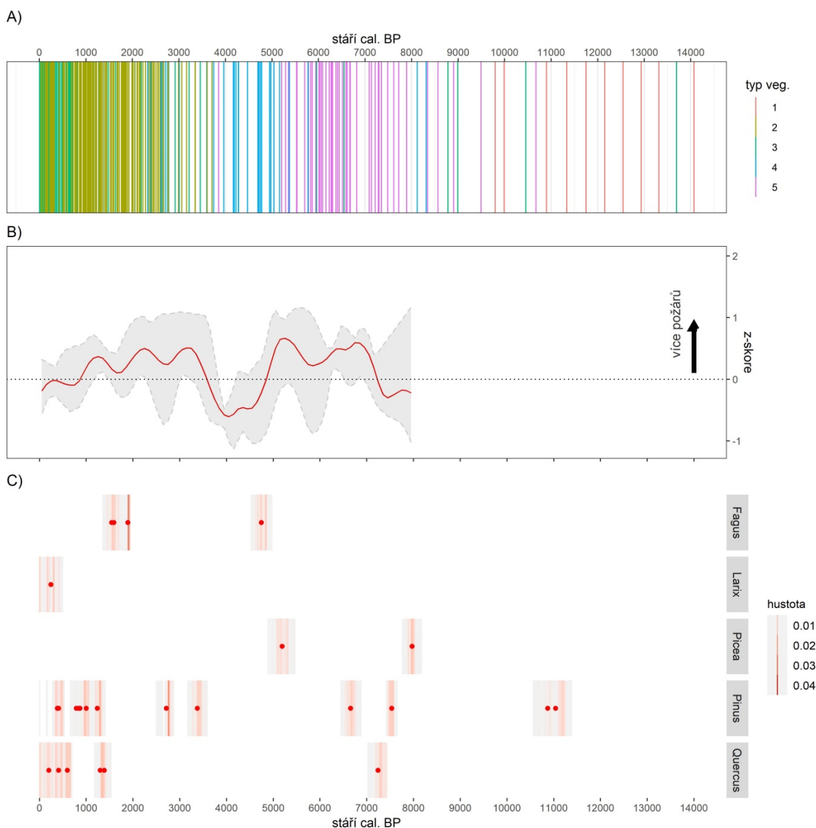
Obr. 5 Syntéza všech publikovaných paleoenviromentálních záznamů holocenního vývoje vegetace a požárového záznamu na území NPCŠ. A) Barevné pruhy znázorňují příslušnost fosilního pylového spektra k určitému vegetačnímu typu. Clust 1 – březo-borové lesy (s výskytem Pinus cembra ), 2- jedlo-bukové lesy, 3- borové lesy, 4- bučiny (období expanze buku), 5- smrkové lesy a smíšené listnaté lesy (dub, jilm, lípa, líska). B) Regionální požárová aktivita odvozená z množství uhlíků v sedimentu. C) Mikroskopicky determinované uhlíky z půdních profilů a jejich stáří stanovené radiokarbonovou metodou. Bod označuje medián kalibrovaného stáří a intenzita červené hustoty pravděpodobnosti v kalibračním intervalu 2 sigma (celý rozsah označen šedě).
