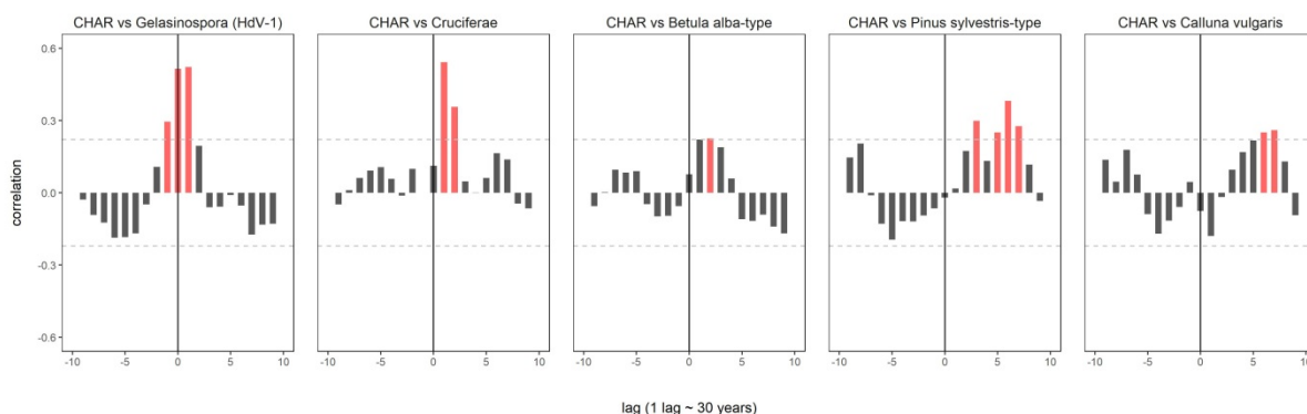
Obr. 8. Sukcesní vývoj po požárech v období 2689-5054 cal BP na lokalitě Velké ohbí v Adršpašských skalách. Cross-korelační analýza mezi uhlíkovým záznamem (CHAR) a vybraných rostlin a hub. Horizontální osa označuje časový odstup po požáru (kladná hodnota lag, 1 lag odpovídá úseku 30 let),
