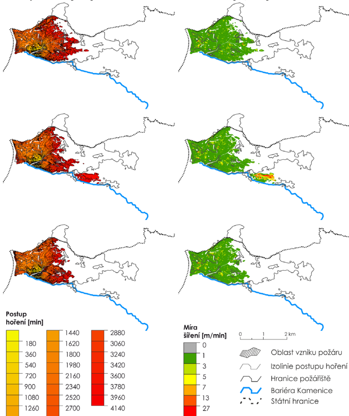
Obr.80 Ukázka tří simulací představující požár ve zdravém smrkovém lese
