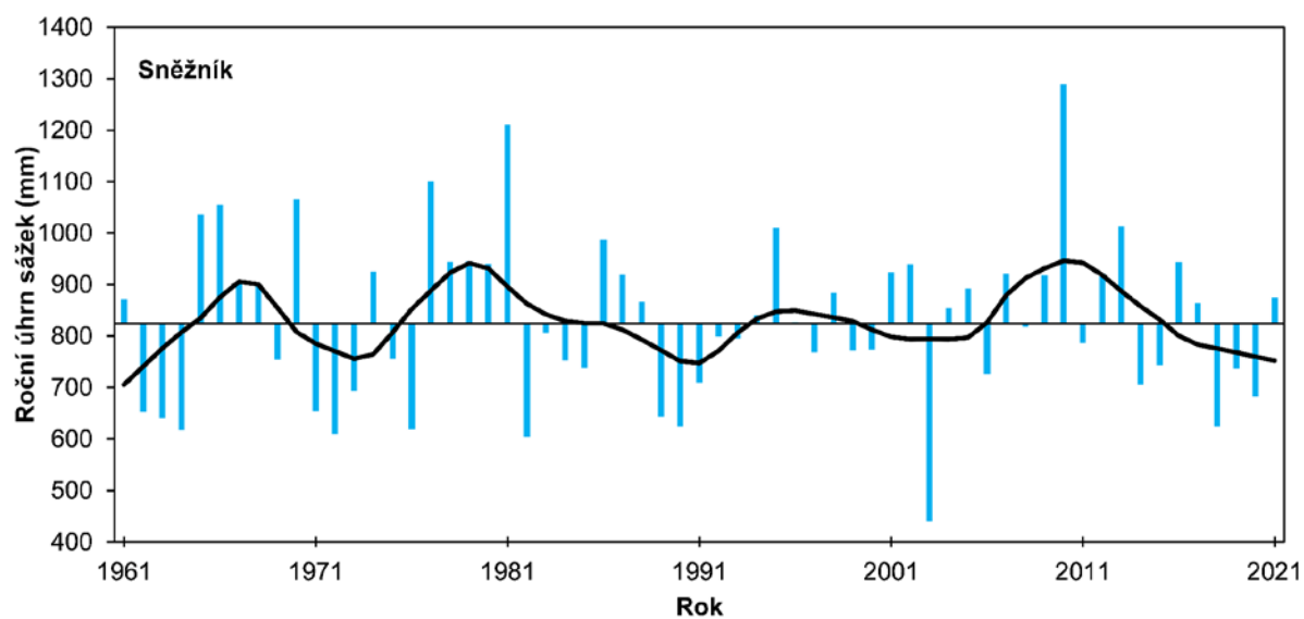
Obr. 41 Kolísání ročních úhrnů srážek vyjádřené odchylkami od normálu 1991 až 2020 na stanicích Děčín a Sněžník. Shlazeno Gaussovým filtrem pro 10 let.
