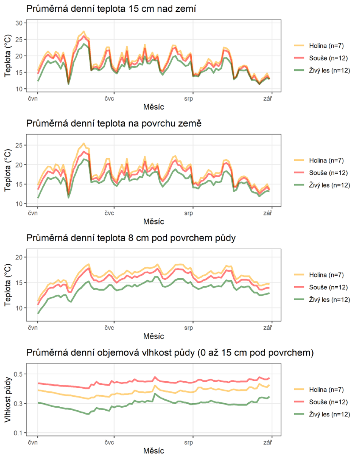
Obr. 9b. Srovnání mikroklimatických podmínek v živých smrkových porostech (živý les), odumřelých smrkových porostech se 100% ponechanými soušemi (souše) a kompletně vytěžených smrkových porostech (holina). Data poskytl Oddělení GIS a DPZ, Botanický ústav AV ČR.
