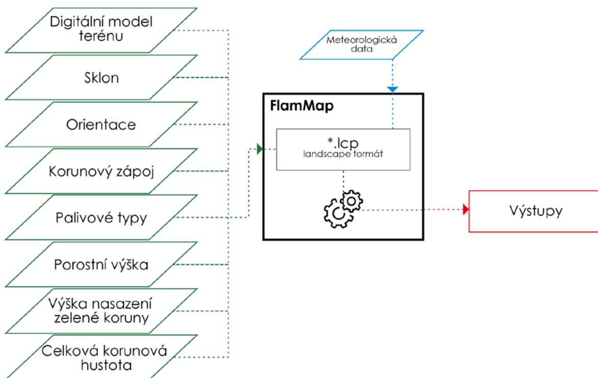
Obr. 66 Vstupní vrstvy do programu FlamMap v rozlišení 5 x 5 m
