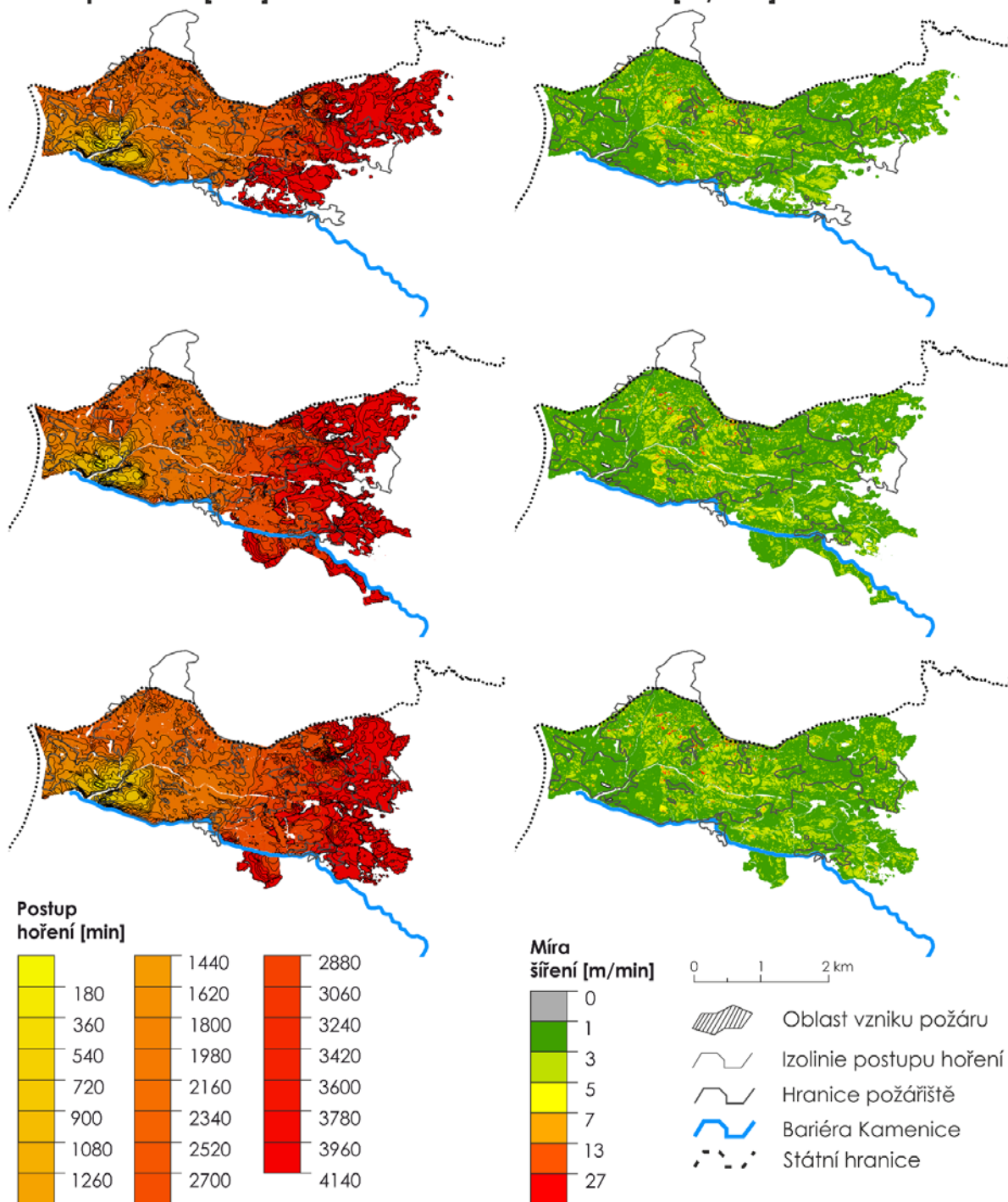
Obr. 71 Ukázka tří simulací reflektující reálný postup požáru za aktuálně dostupných informací, a to na příkladu charakteristiky požáru Postup hoření a Míry šíření
