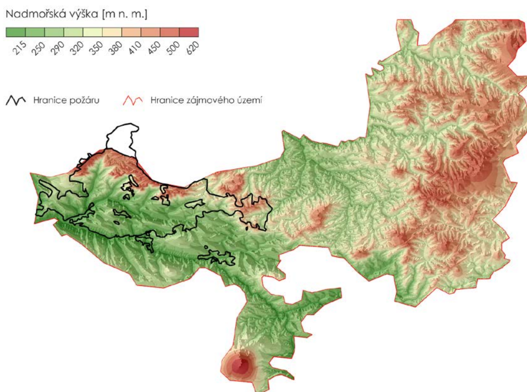
Obr. 67 Vstupní vrstva do programu FlamMap v rozlišení 5 x 5 m, digitální model terénu
