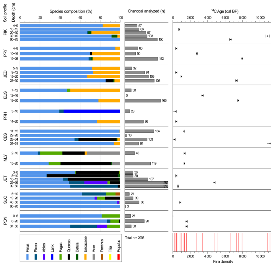
Obr. 9 Druhové složení uhlíkových spekter v půdních sondách z území NPČŠ. Převzato z publikace (Bobek et al., 2018).
