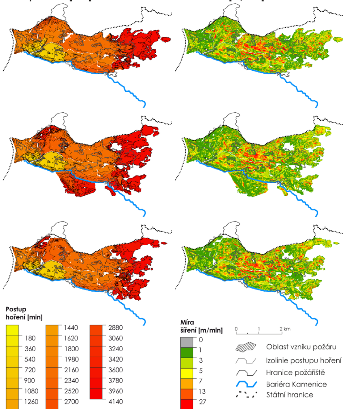
Obr. 83 Ukázka tří simulací představující požár v holínách, Postup hoření a Míra šíření
