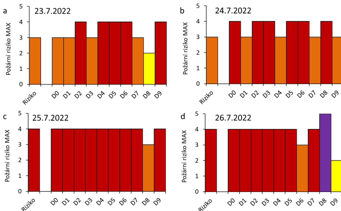
Obr. 63 Předpověď maximální požární riziko (souhrnný index) pro zkoumanou oblast na období počátku požáru (23–26.7.2022) – riziko (skutečnost), předpověď na daný den (D0) až 9 dnů dopředu (D9)
