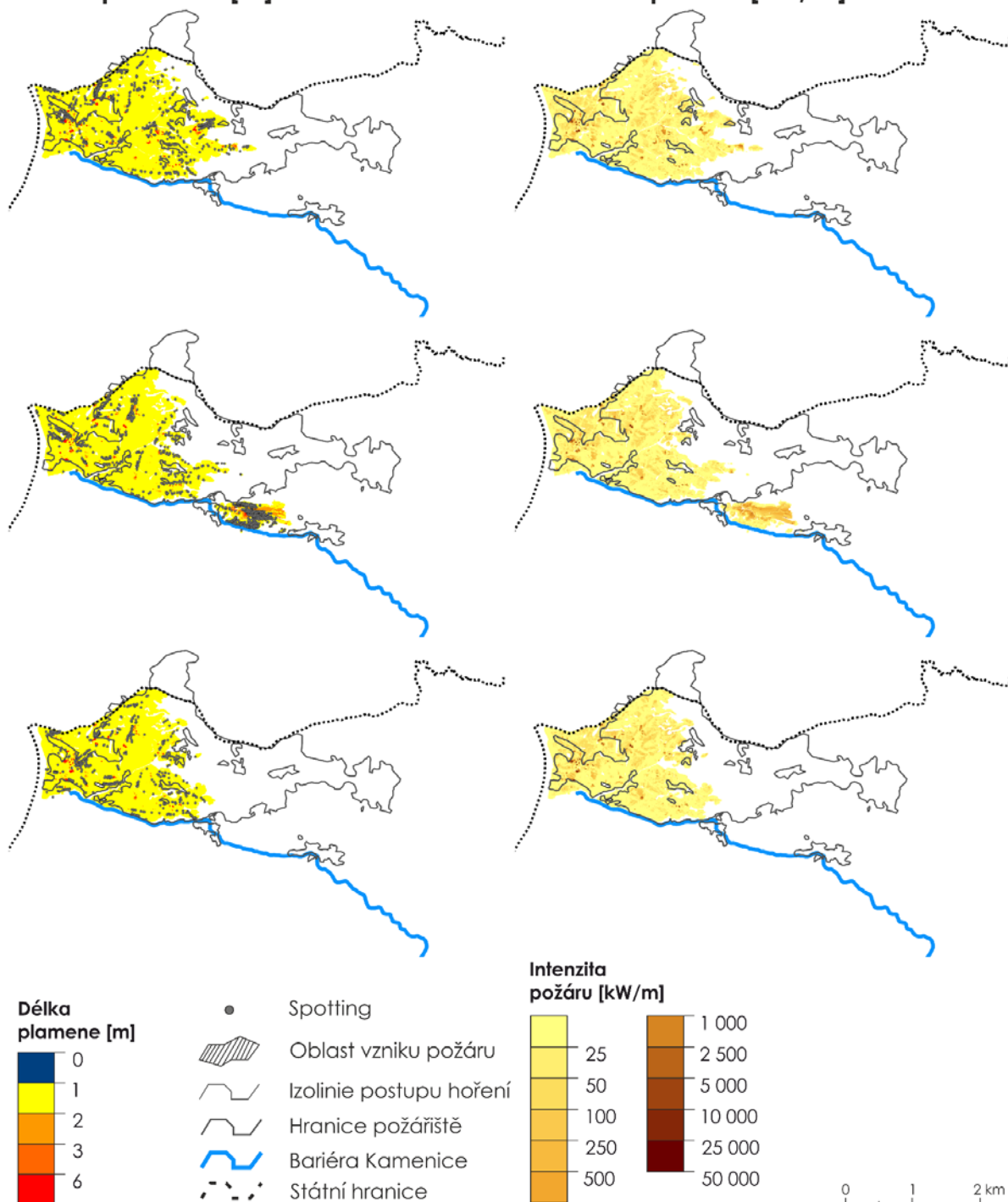
Obr.81 Ukázka tří simulací představující požár ve zdravém smrkovém lese
