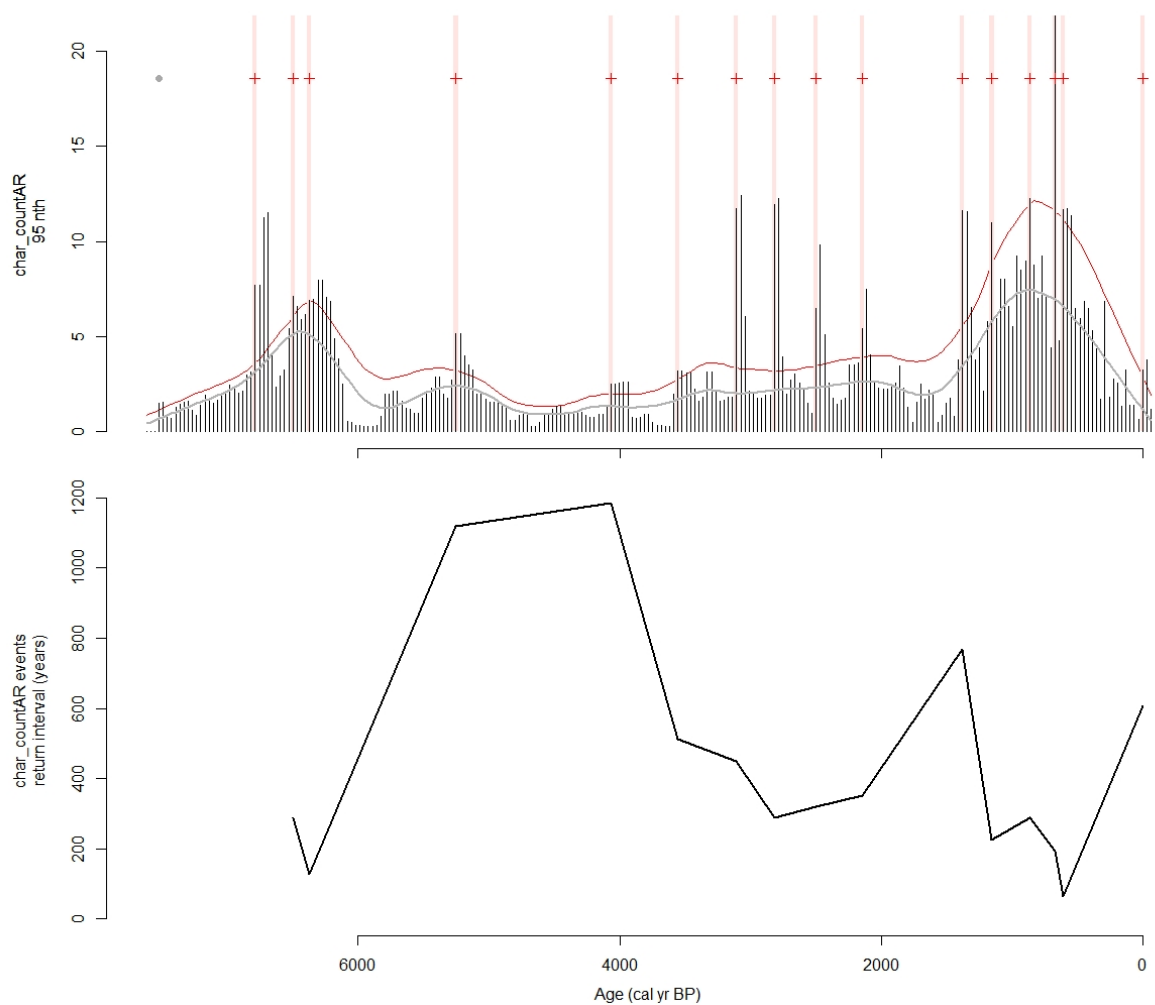
Obr. 6 Požárová historie na lokalitě Eustach. Horní panel – sloupkový graf množství depozice uhlíků do sedimentu (CHAR), červená křivka představuje dlouhodobý trend, křížky označují statisticky významné požárové události. Spodní panel – interval návratu požáru (fire return interval, FRI). Převzato z publikace (Bobek et al., 2018).
