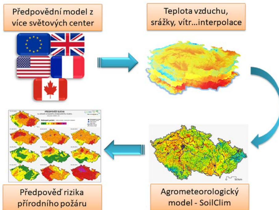
Obr. 58 Schéma přípravy předpovědi rizika přírodního požáru
