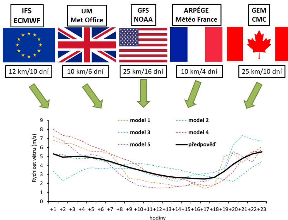
Obr. 57 Schéma použitých modelů, jejich rozlišení, délka předpovědi a princip rozdílných výstupů a tvorba nejpravděpodobnějšího vývoje počasí v dalších hodinách.
