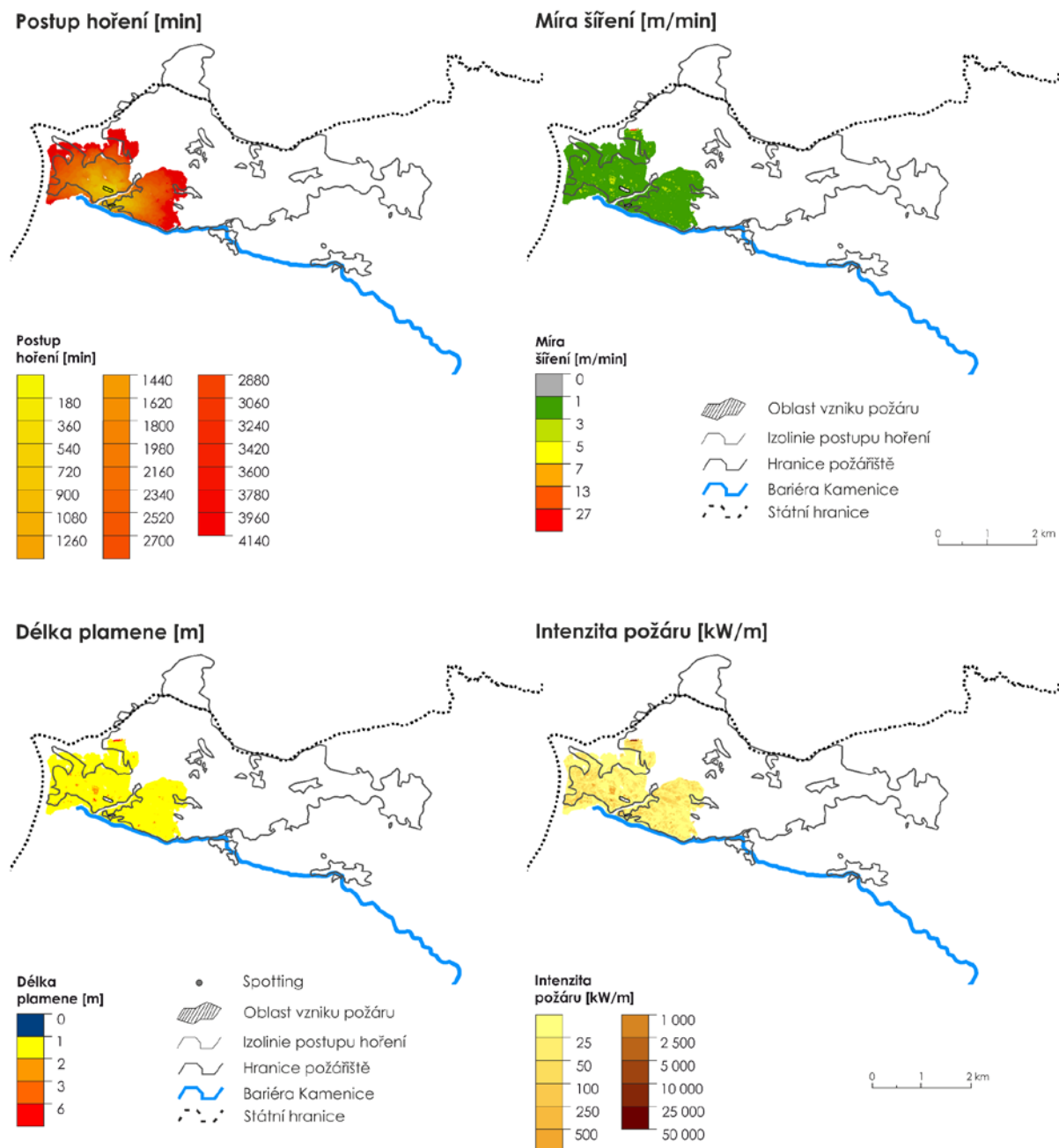
Obr. 73 Postup hoření a míra šíření za změněných podmínek větru (průměrná rychlost a příslušný směr na meteorologické stanici Tokáň)
