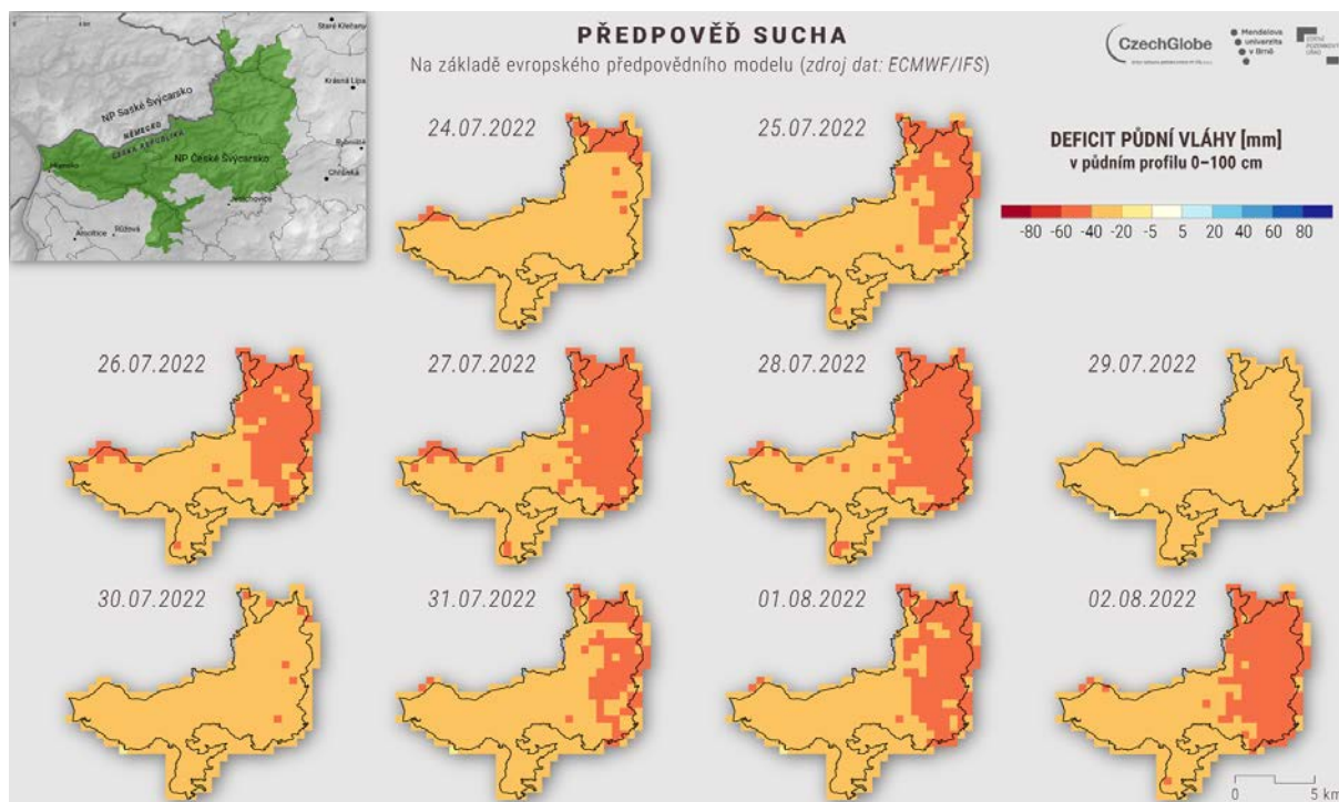
Obr. 55 Zachycuje anomálii půdní vlhkosti v mm oproti obvyklému stavu v daném období v roce v období vzniku a intenzivního šíření požáru na území NP České Švýcarsko podle dat portálu Intersucho.cz a FireRik.cz.
