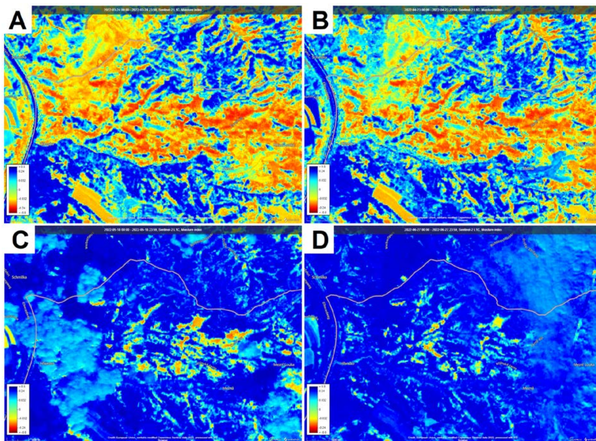
Obr. 50 Vlhkostní index získaný družicí Sentinel 2 dne 24. března 2022 (A), 23. dubna 2022 (B), 18. května 2022 (C) a 27. června 2022 (D).
