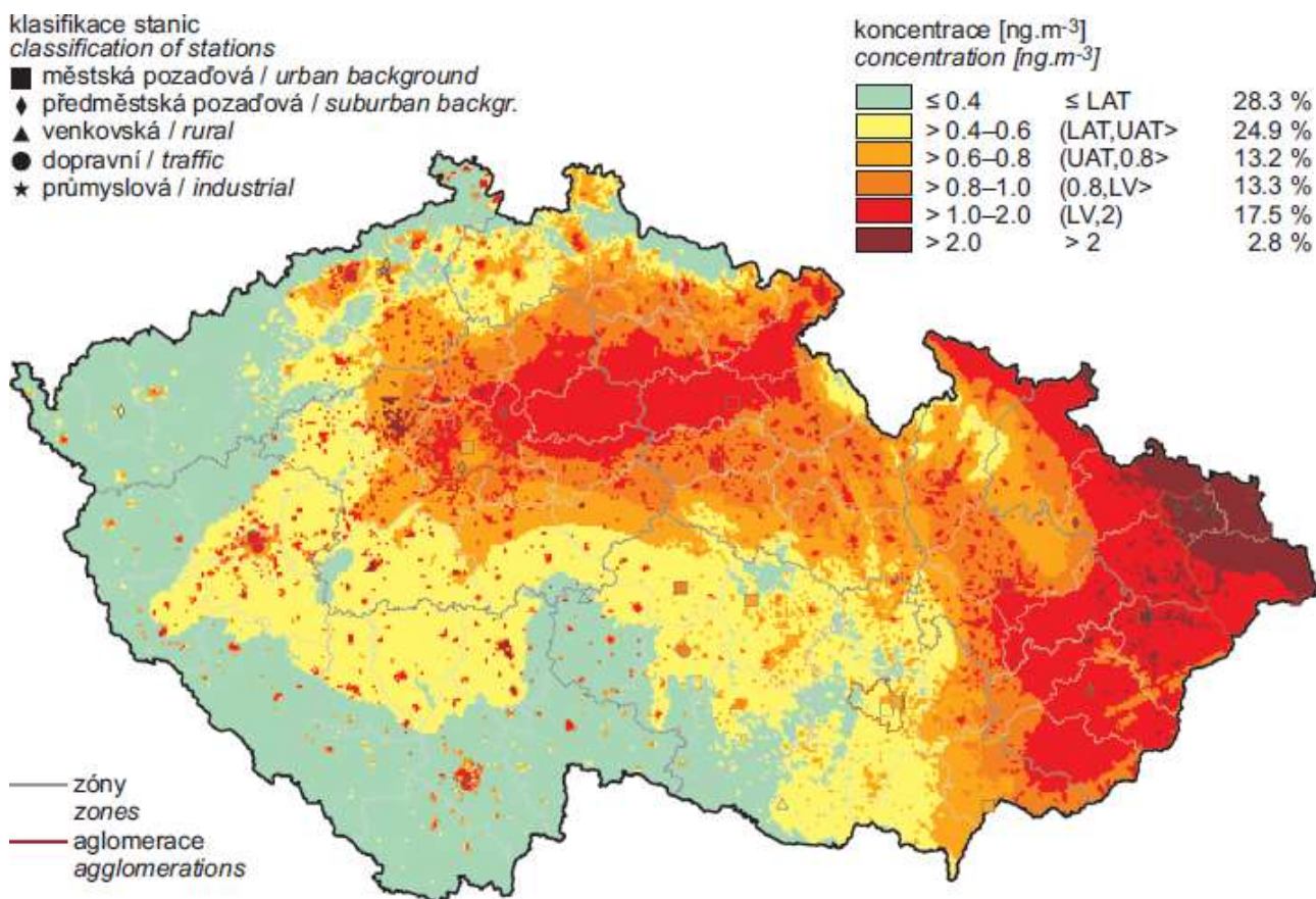
Obr. 20 Pole roční průměrné koncentrace benzo[a]pyrenu v ovzduší v roce 2015
