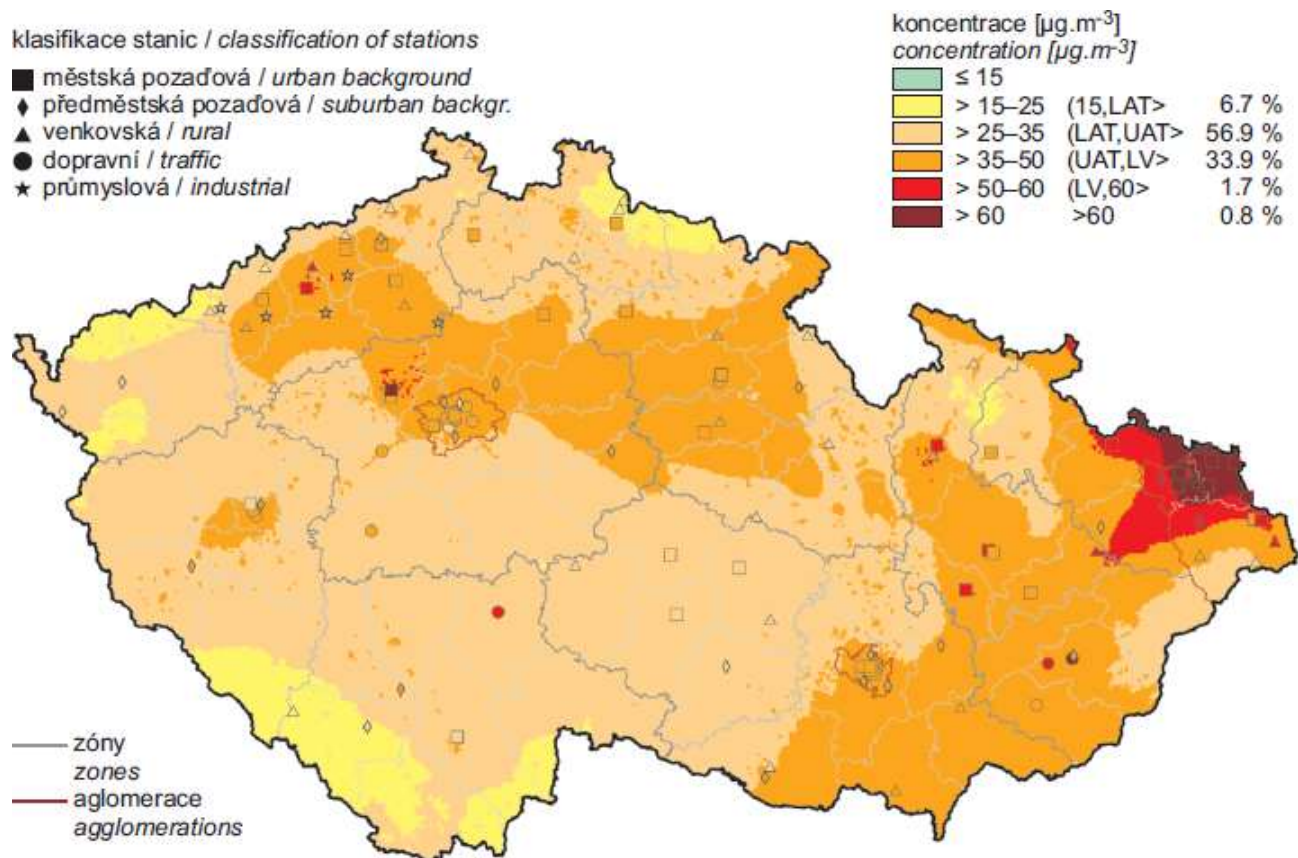
Obr. 15 Pole 36. nejvyšší 24hod. koncentrace \text{PM}_{10} v roce 2015
