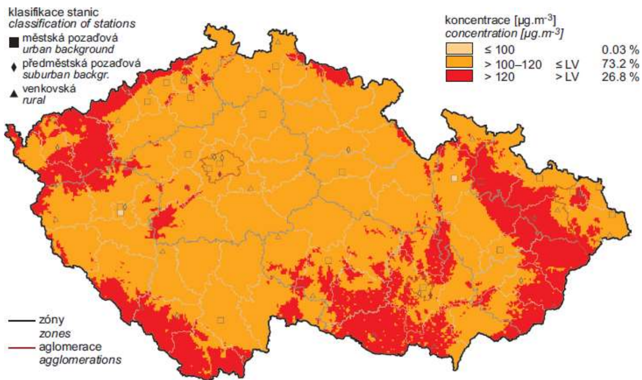
Obr. 21 Pole 26. nejvyššího maximálního denního 8hod. klouzavého průměru koncentrace přízemního ozonu v průměru za 3 roky, 2013–2015
