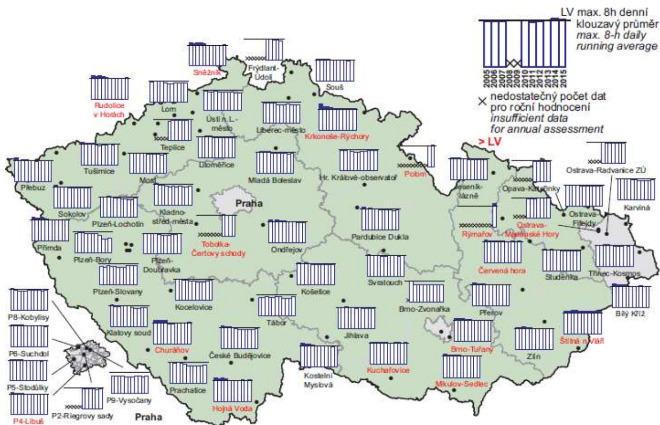
Obr. 13 26. nejvyšší hodnoty maximálního denního 8hod. klouzavého průměru koncentrací přízemního ozonu v průměru za 3 roky v letech 2005–2015 na vybraných stanicích
