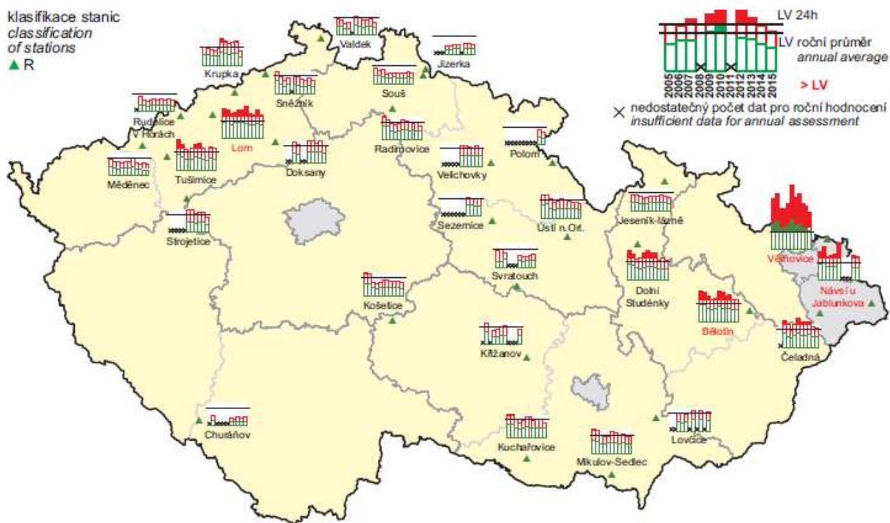
Obr. 4 36. nejvyšší 24hod. koncentrace a roční průměrné koncentrace PM_{10} v letech 2005–2015 na vybraných venkovských (R) stanicích
