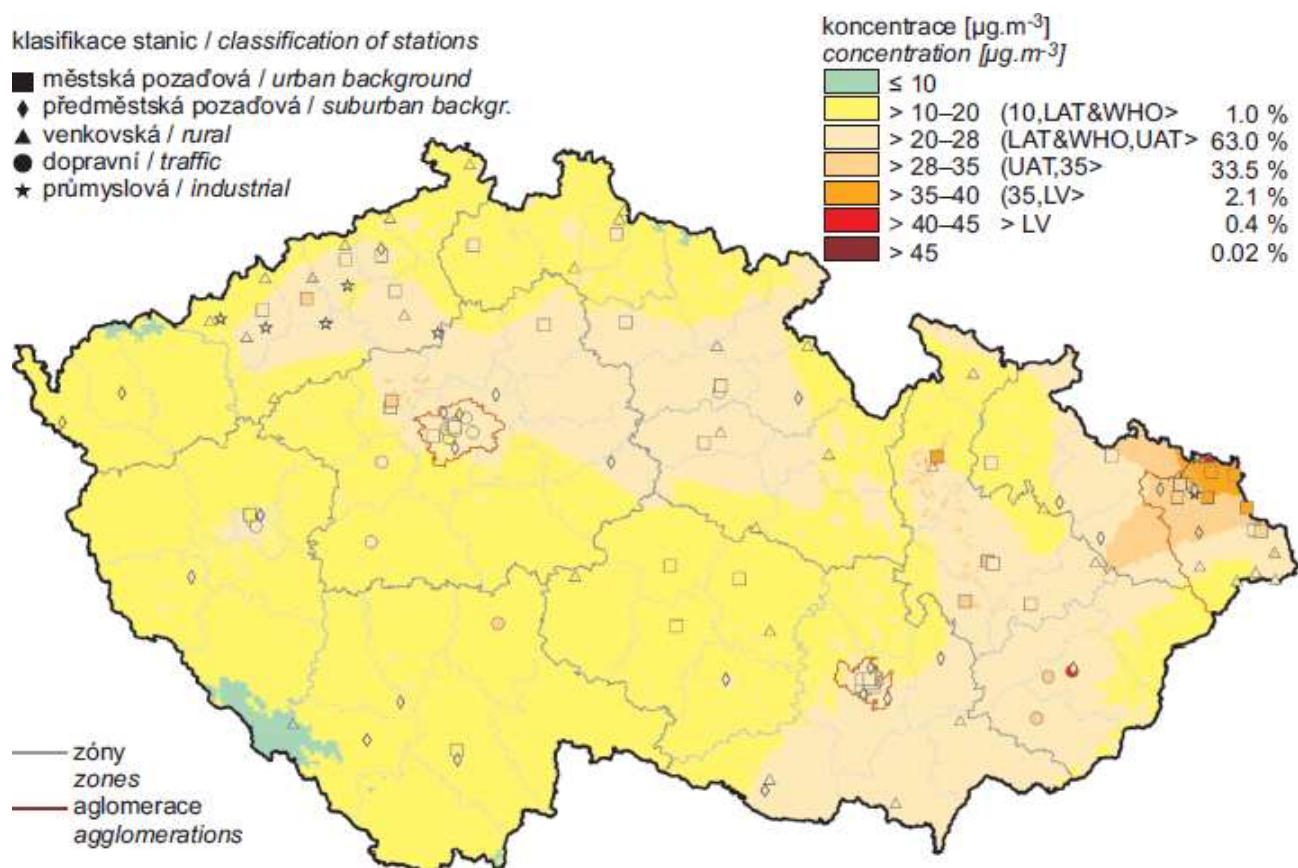
Obr. 16 Pole roční průměrné koncentrace \text{PM}_{10} v roce 2015
