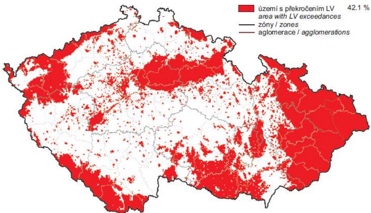
Obr. 23 Vyznačení oblastí s překročenými imisními limity pro ochranu zdraví se zahrnutím přízemního ozonu, 2015
