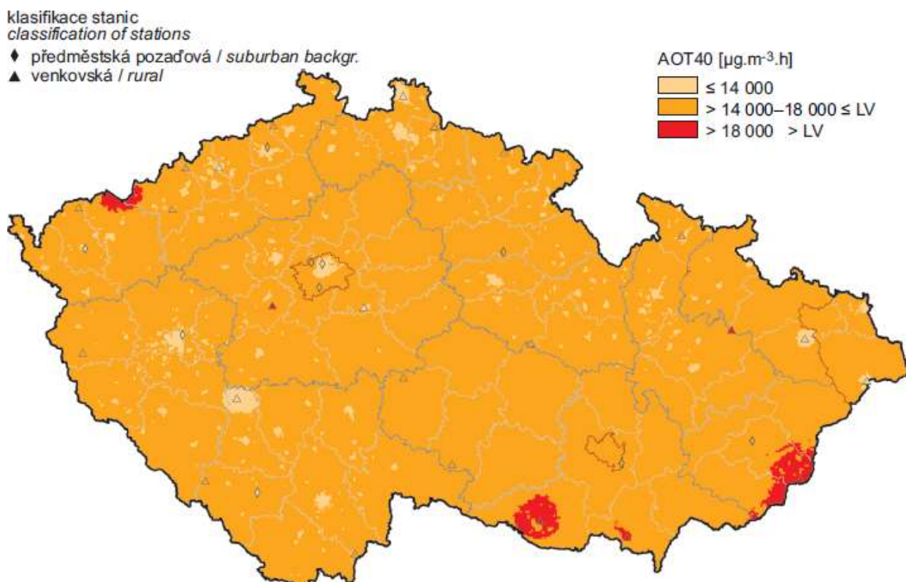
Obr. 22 Pole hodnot expozičního indexu AOT40, průměr za 5 let, 2011–2015
