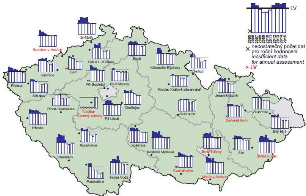
Obr. 14 Hodnoty expozičního indexu AOT40 ozonu v letech 2005–2015 na vybraných stanicích, průměr za 5 let
