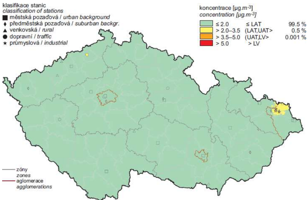
Obr. 19 Pole roční průměrné koncentrace benzenu v ovzduší v roce 2015
