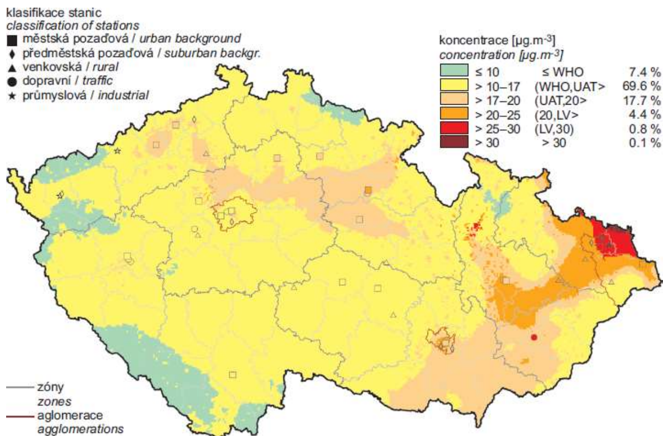
Obr. 17 Pole roční průměrné koncentrace \text{PM}_{2.5} v roce 2015
