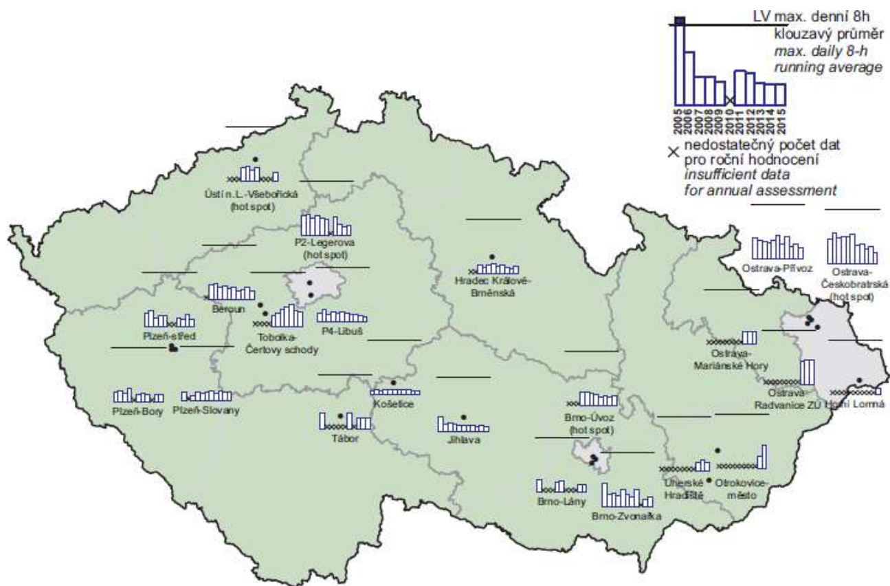
Obr. 7 Maximální denní 8hod. klouzavé průměrné koncentrace CO v letech 2005–2015 na vybraných stanicích
