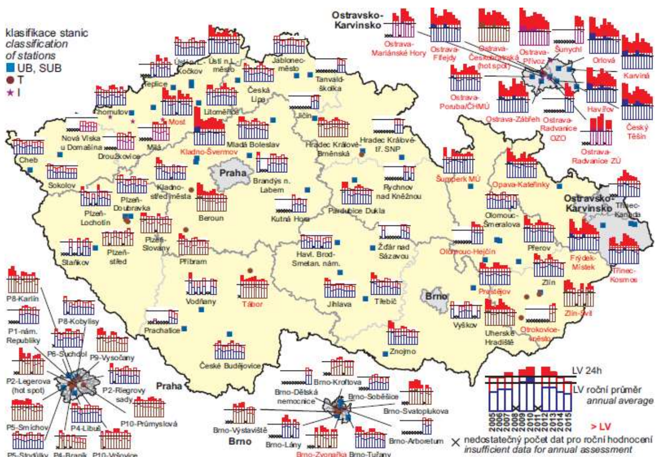
Obr. 3 36. nejvyšší 24hod. koncentrace a roční průměrné koncentrace PM_{10} v letech 2005–2015 na vybraných stanicích s klasifikací UB, SUB, I a T
