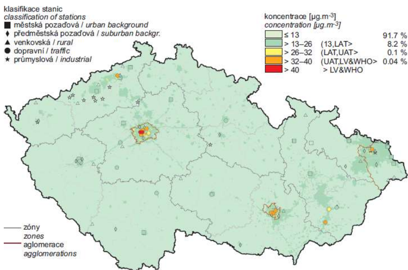
Obr. 18 Pole roční průměrné koncentrace \text{NO}_2 v roce 2015
