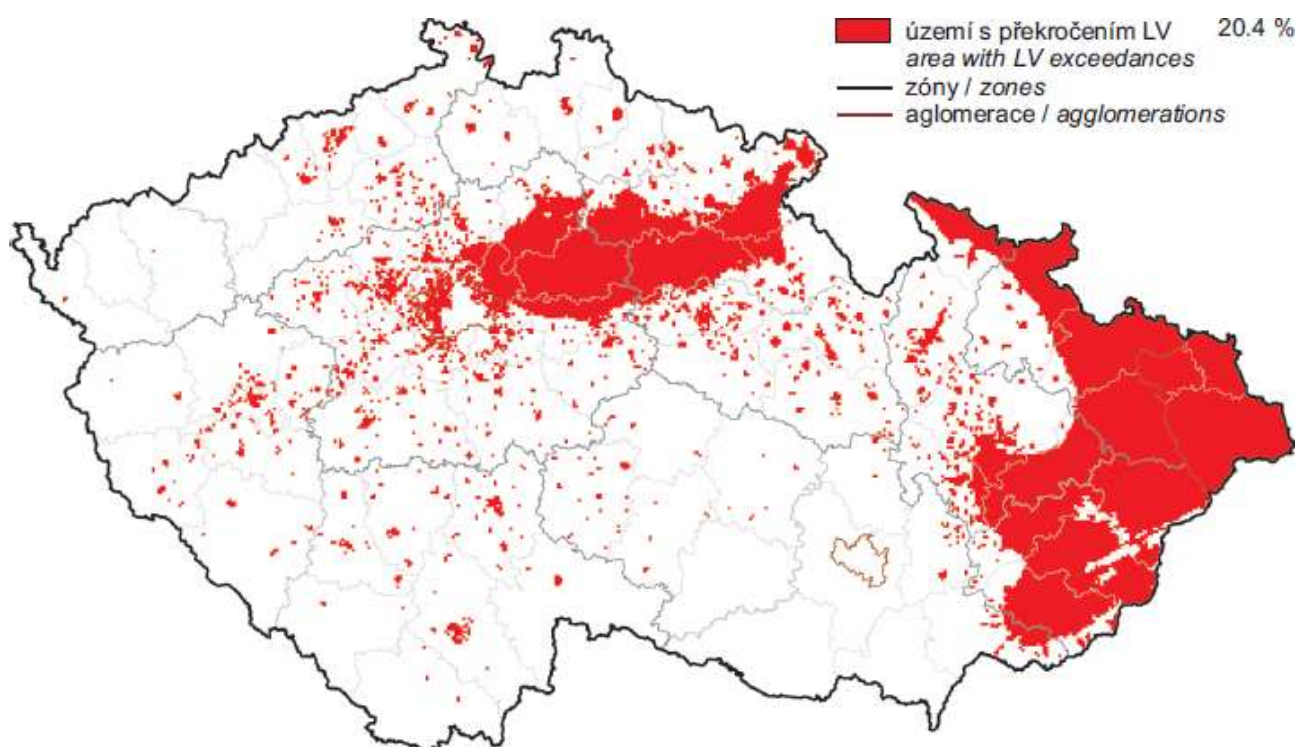
Obr. 24 Vyznačení oblastí s překročenými imisními limity pro ochranu zdraví bez zahrnutí přízemního ozonu, 2015
